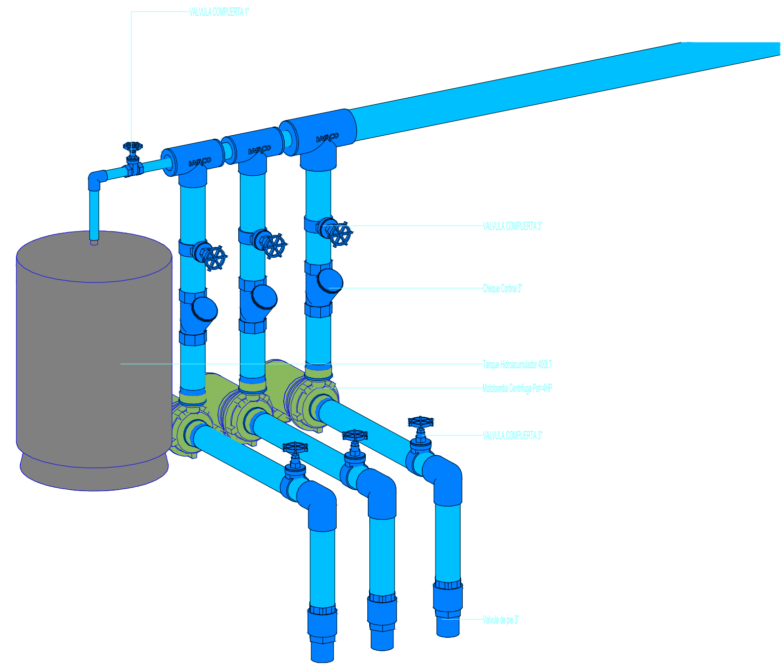
2 ISOMETRIA DETALLE TANQUE SUBTERRANEO - EQUIPOS Esc.: 1 - 10
