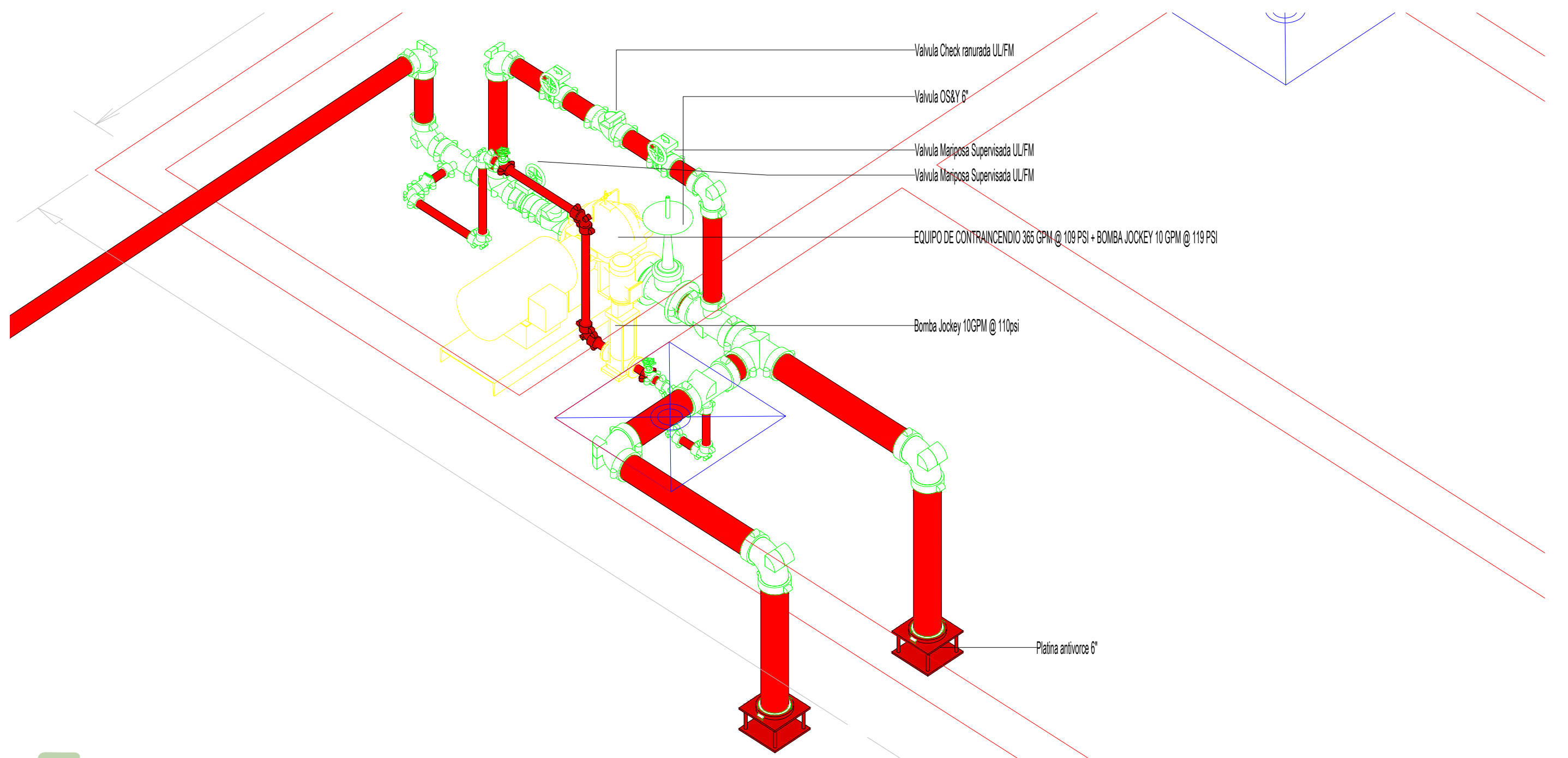
2 DETALLES TANQUE Esc.: SIN ESCALA
