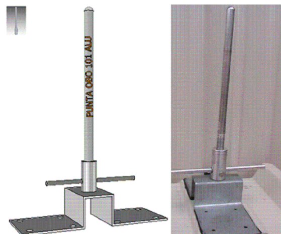
DETALLE N°11 PLATINA AUXILIAR PARA ANCLAR PUNTA OBO EN CUBIERTAS PLANAS SIN PERFORAR CUBIERTA
