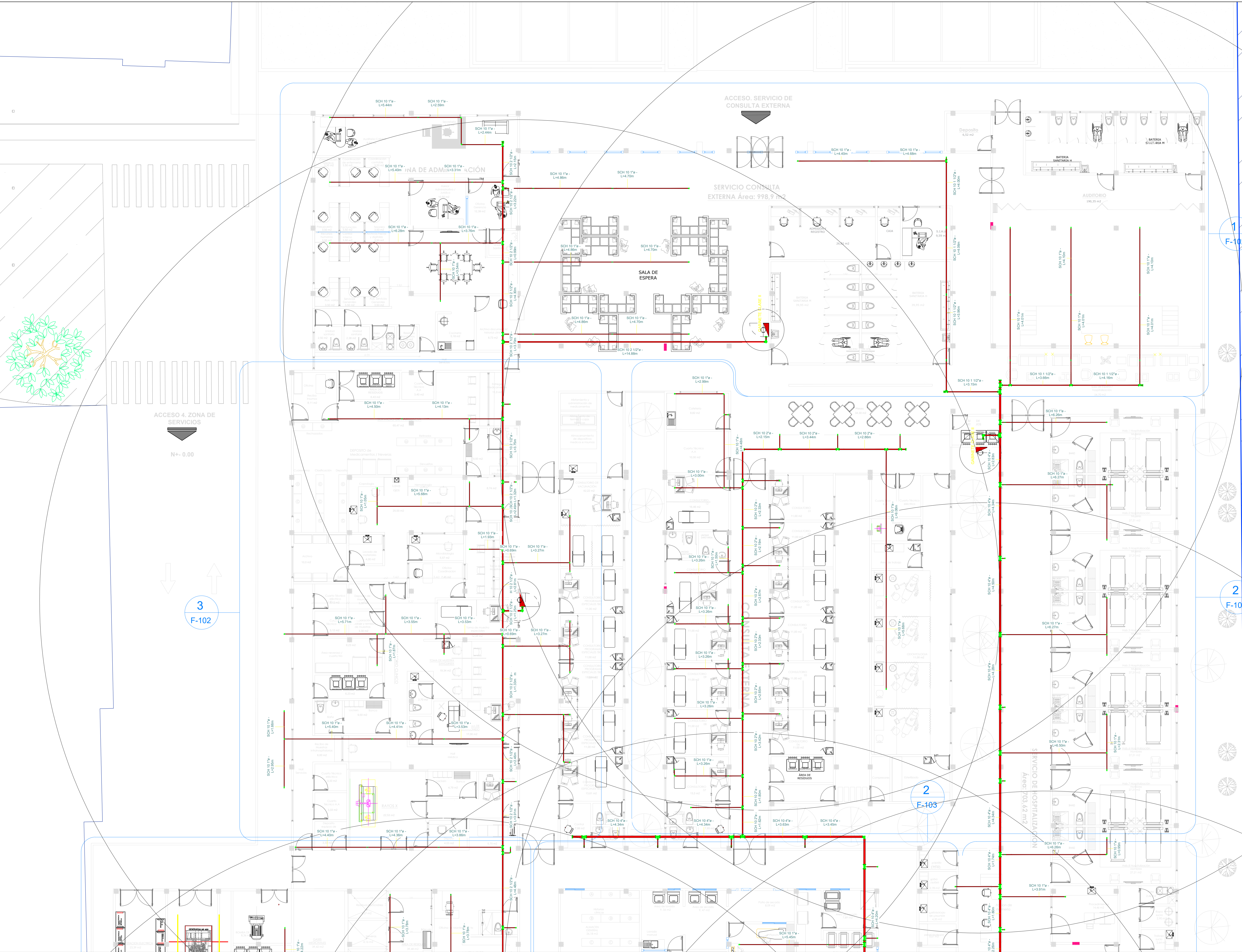
1 SISTEMA DE EXTINCIÓN DE INCENDIOS - AMPLIAICÓN 1 Esc.: 1 : 100
