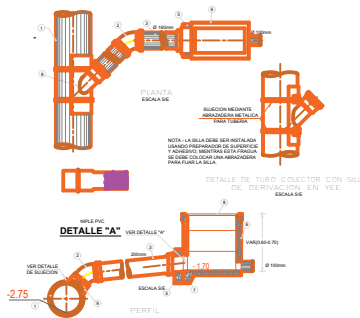
DETALLE DE CONEXION DOMICILIARIA DE DESAGUE
