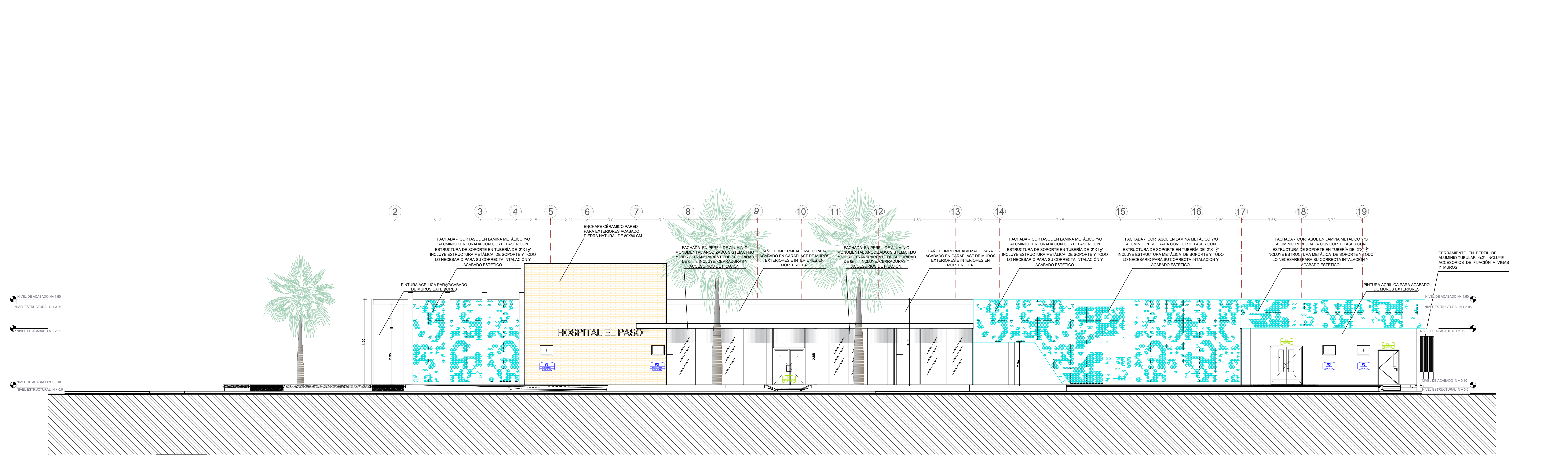
FACHADA FRONTAL- ACCESO URGENCIAS
