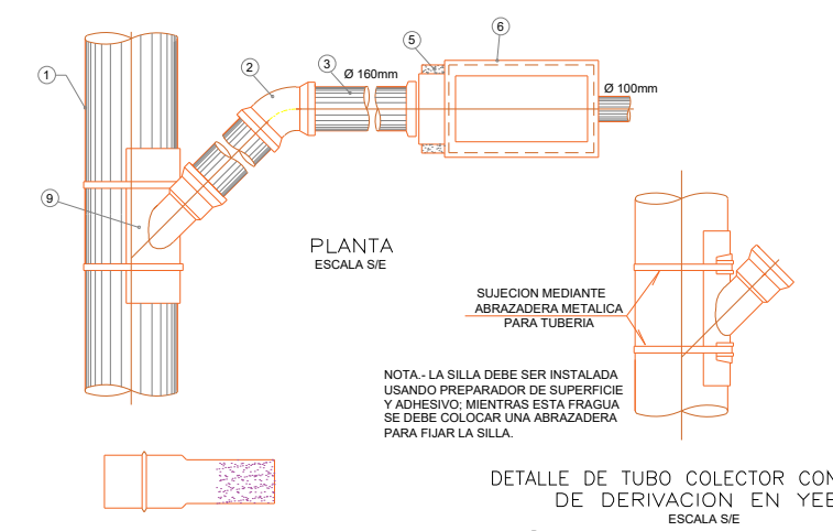
DETALLE DE CONEXION DOMICILIARIA DE DESAGUE
