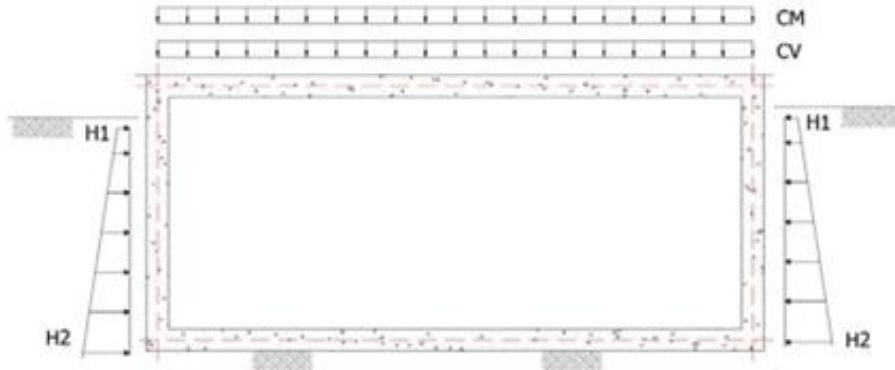
Cargas actuantes en la estructura
