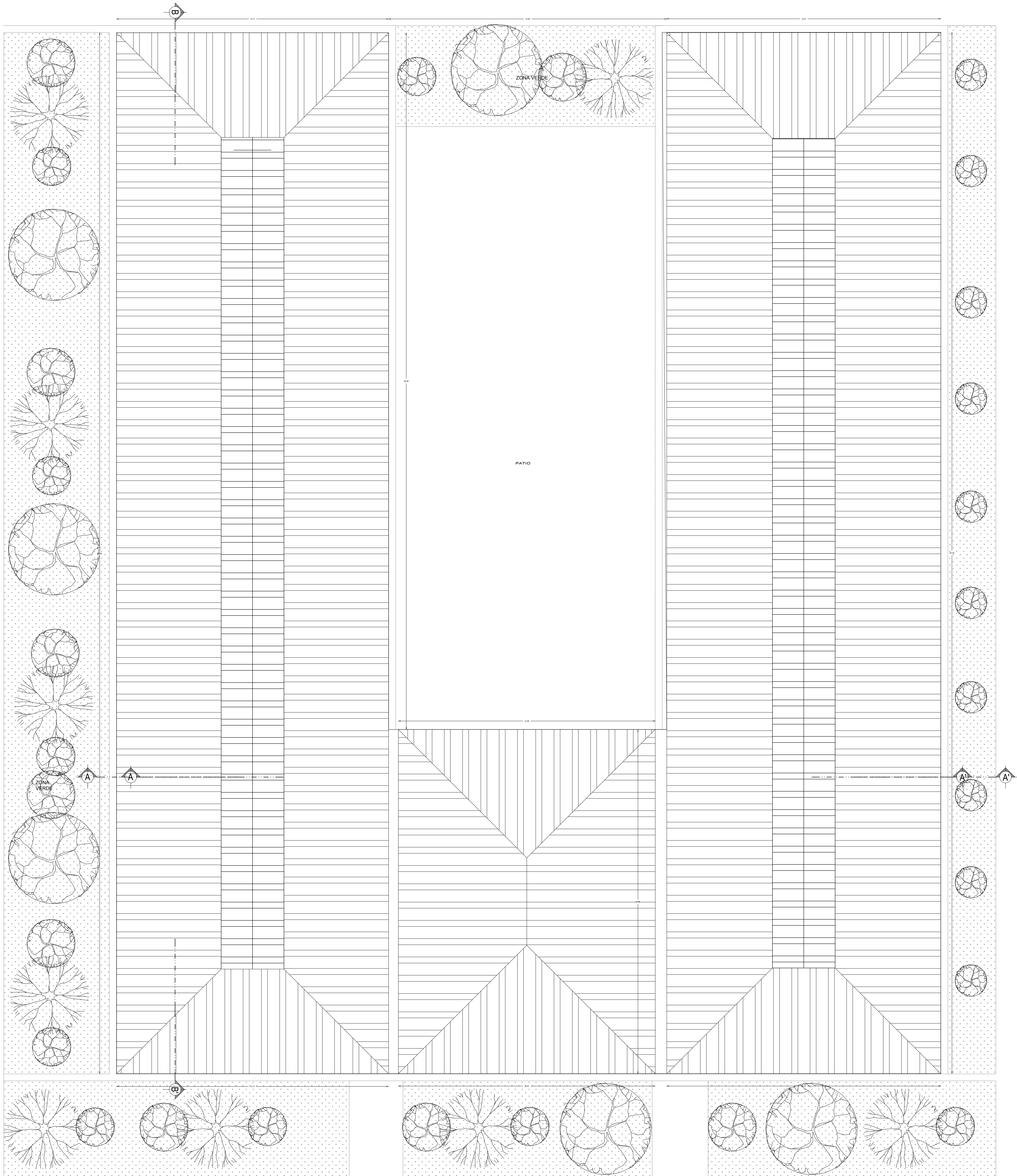
PLANTA DE CUBIERTA ESCALA 1:100
