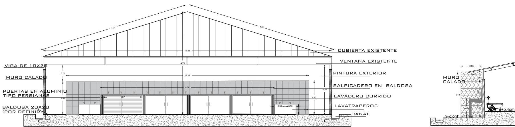
FACHADA LAVADERO ESCALA 1:100
