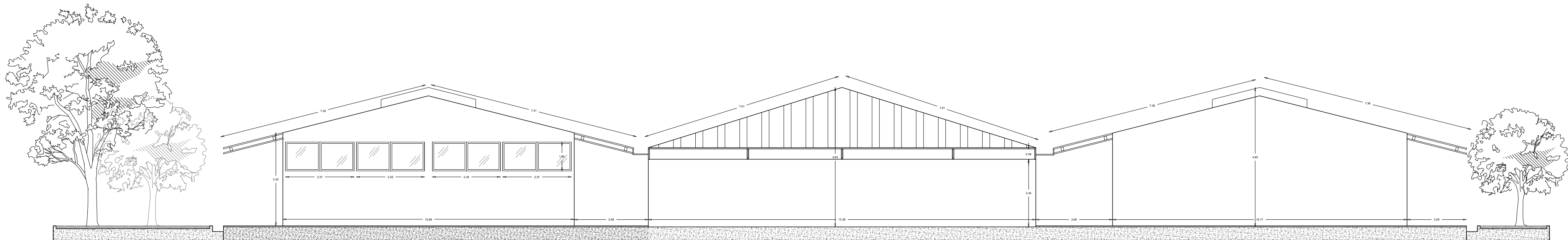
FACHADA ESCALA 1:100
