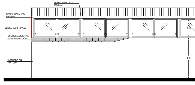
DETALLE 01 ESCALA 1:100
