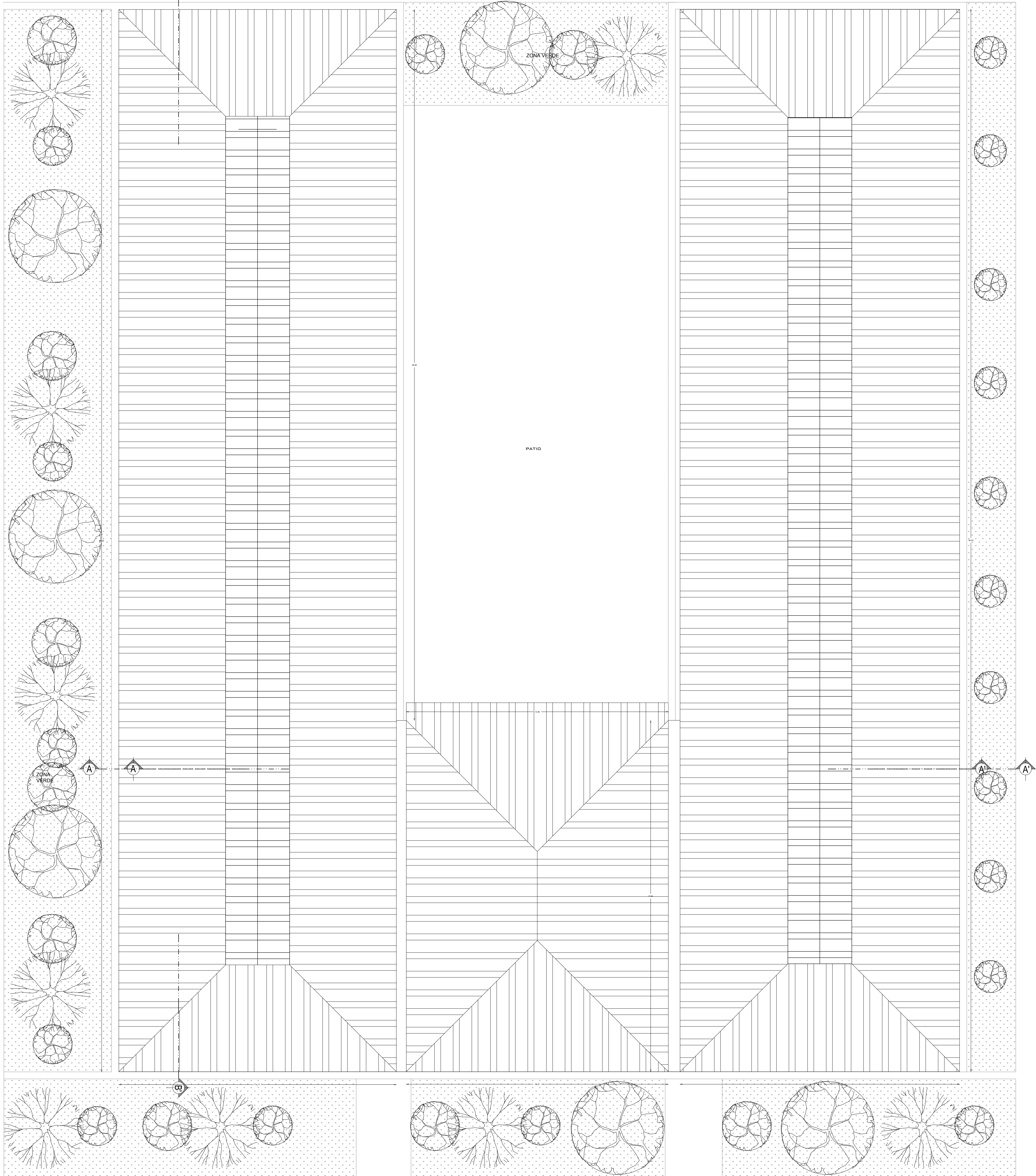
PLANTA DE CUBIERTA ESCALA 1:100
