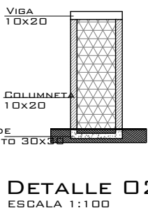
DETALLE 02 ESCALA 1:100
