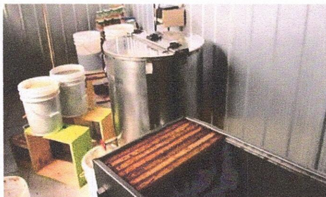
Sistema de extracción de miel.
