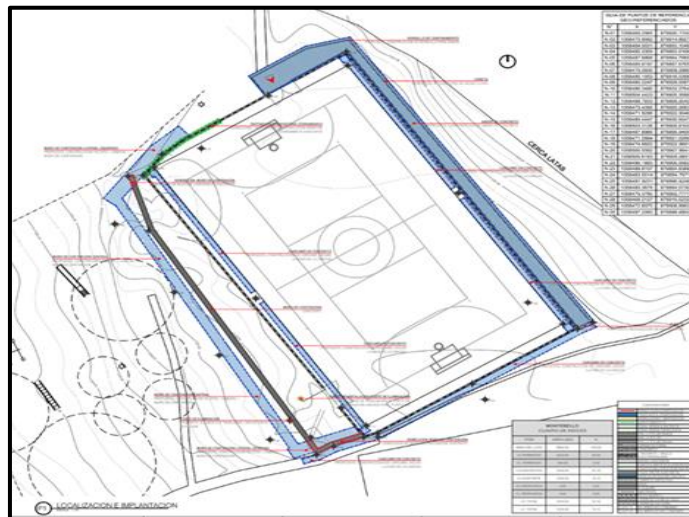
GRÁFICA 19: Planta General de implantación escenario cancha múltiple Montebello.
