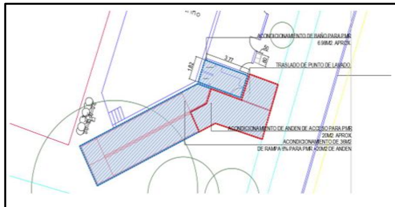
GRÁFICA 20: Planta General de implantación escenario deportivo el Guabal.
