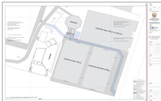
GRÁFICA 23:Planta General de implantación escenario deportivo La Selva.
