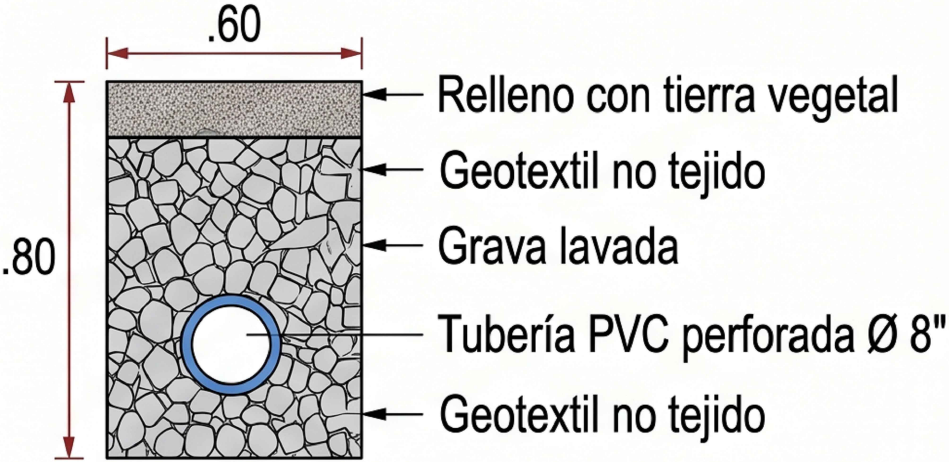
DETALLE CAMPO DE INFILTRACIÓN (Sección típica)
