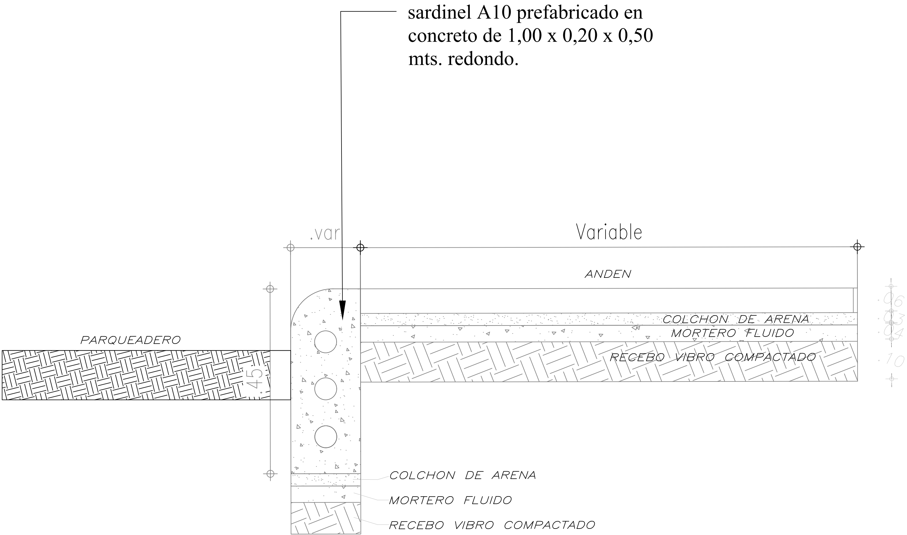
DETALLE SARDINEL Escala 1 : 10
