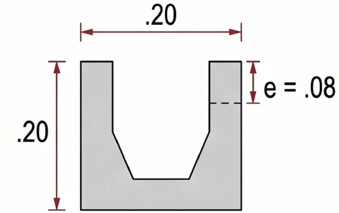
DETALLE CUNETA PERIMETRAL (0,20 x 0,20 m)
