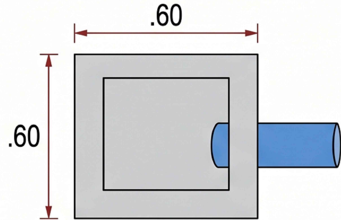
DETALLE CAJA DE INSPECCIÓN (0,60 x 0,60 x 0,60 m)
