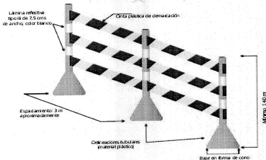
Ilustración 8: Banderines Tubulares
