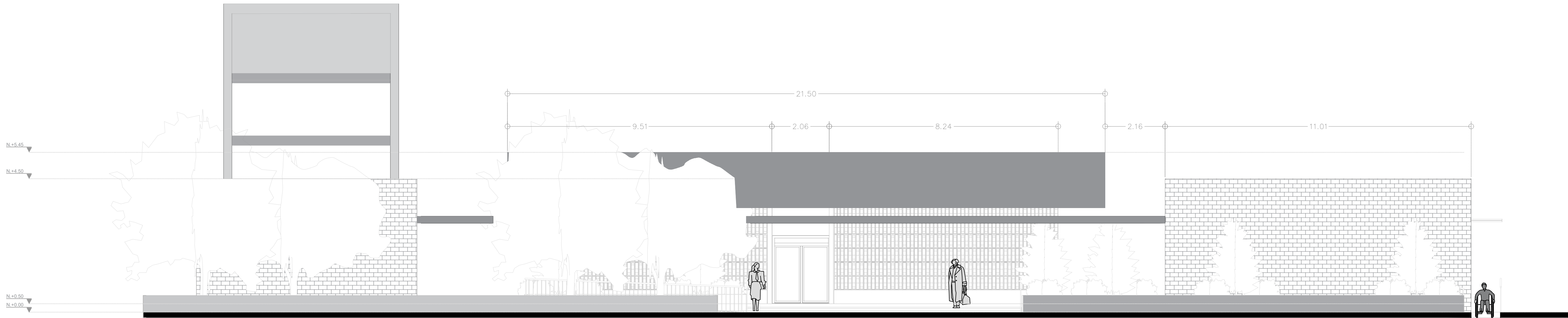
FACHADA NORTE CENTRO VIDA .....Esc:1/75
