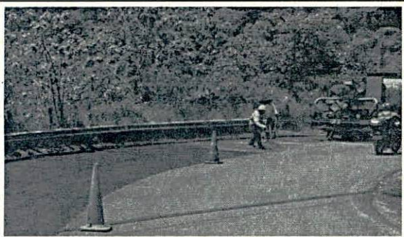
DESCRIPCIÓN: Riego de liga.
