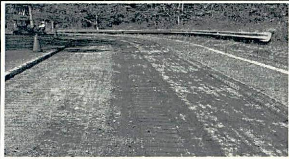
DESCRIPCIÓN: Demolición y fresado de carpeta existente.
