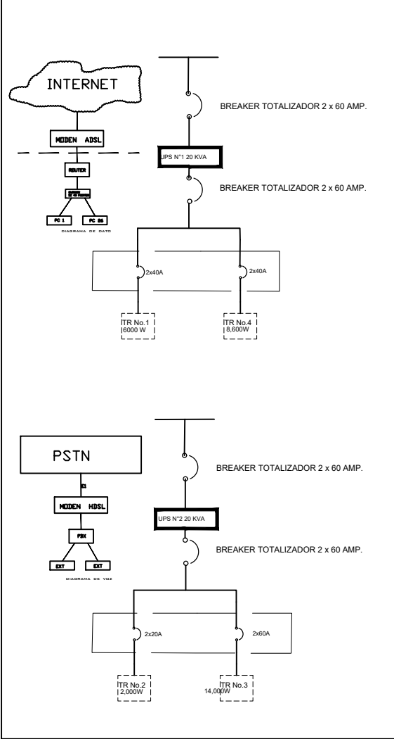
DIAGRAMA UNIFILAR TABLEROS REGULADO
