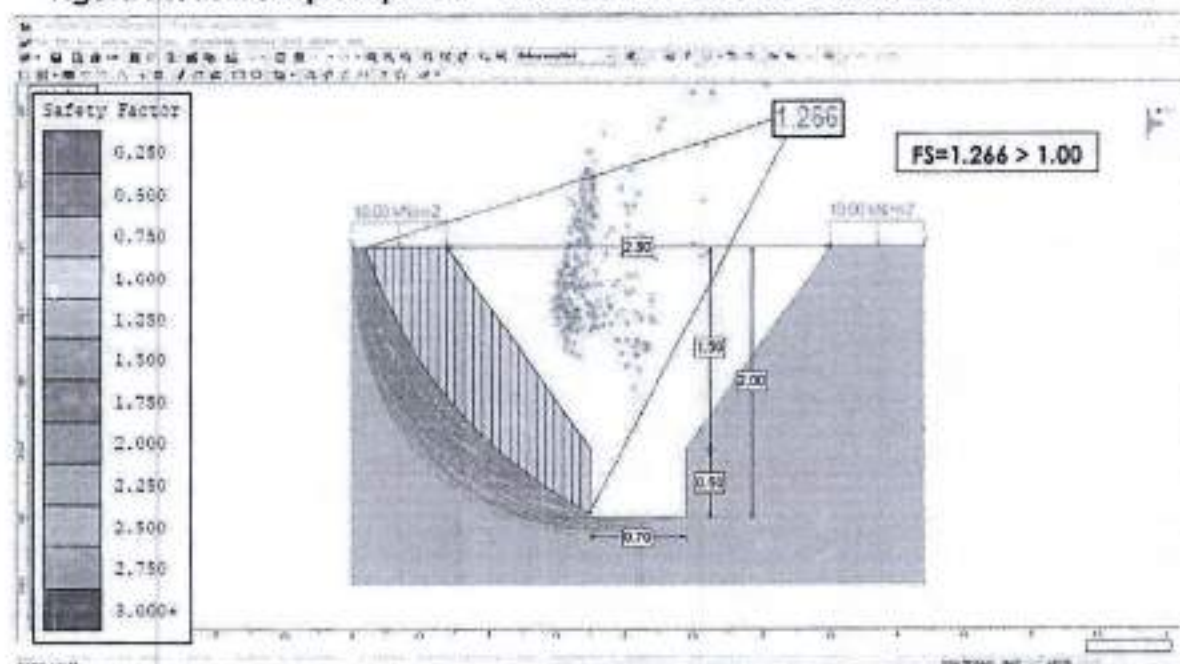
Figura 26. FS Bishop simplified – Excavación colector talud 0.70H:1V con sismo
