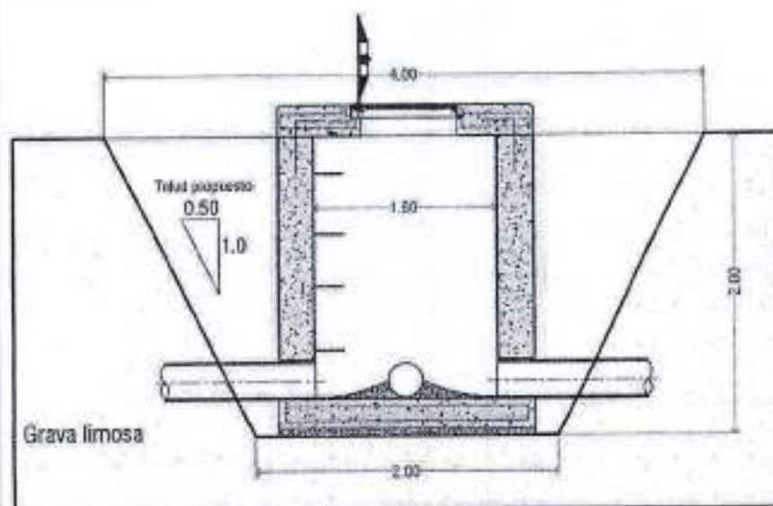
Figura 10. Creación del modelo en Autocad excavación para pozos
