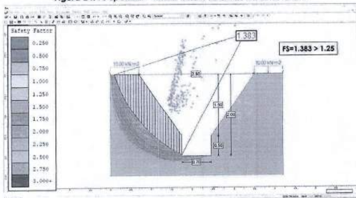
Figura 24. FS Spencer – Excavación colector talud 0.70H:1V
