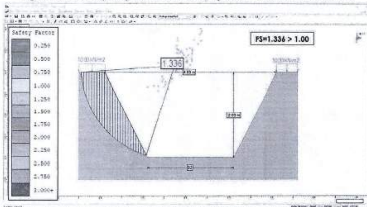
Figura 19. FS Bishop simplified – Excavación pozos talud 0.5H:1V con sismo
