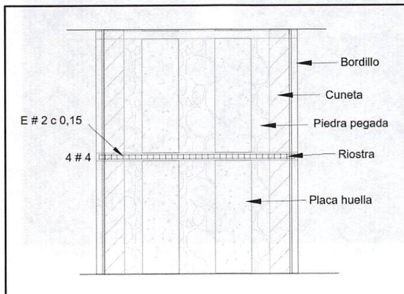
Figura 2.4 Planta
