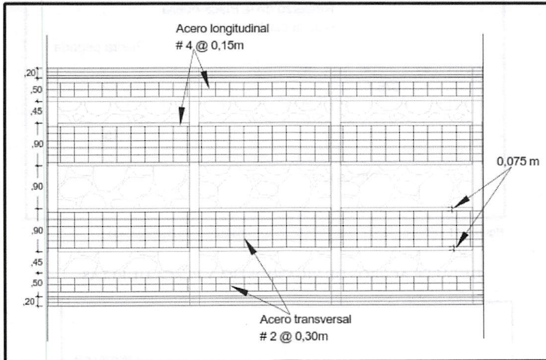
Figura 2.1 Planta de Distribución del refuerzo
