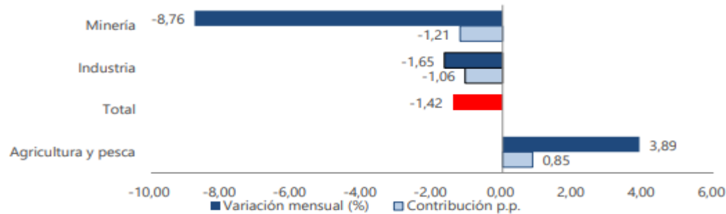
Gráfico 2. Variación y contribución mensual del IPP de Producción Nacional por secciones CIU Rev.4.0 A.C Julio 2026pr
