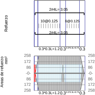
VCP8 / Base F´c=21Mpa Fy=420Mpa d'=60mm
