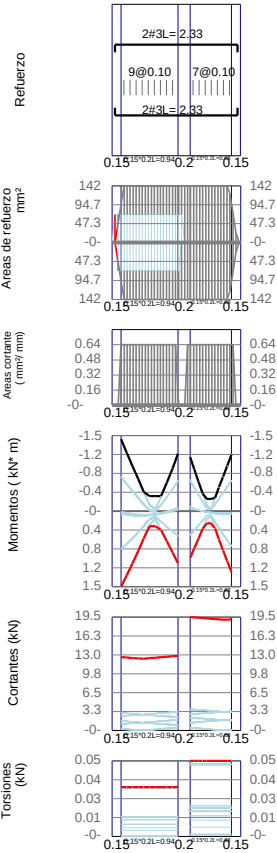
VP3 / Story1 F´c=21Mpa Fy=420Mpa d'=60mm
