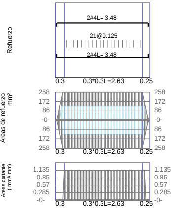
VCP6 / Base F'c=21\text{Mpa} Fy=420\text{Mpa} d'=60\text{mm}
