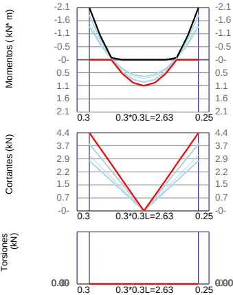
VCP7 / Base F´c=21Mpa Fy=420Mpa d'=60mm
