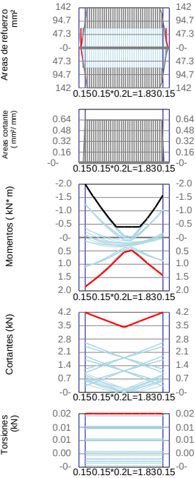
VP2 / Story1 F´c=21Mpa Fy=420Mpa d'=60mm
