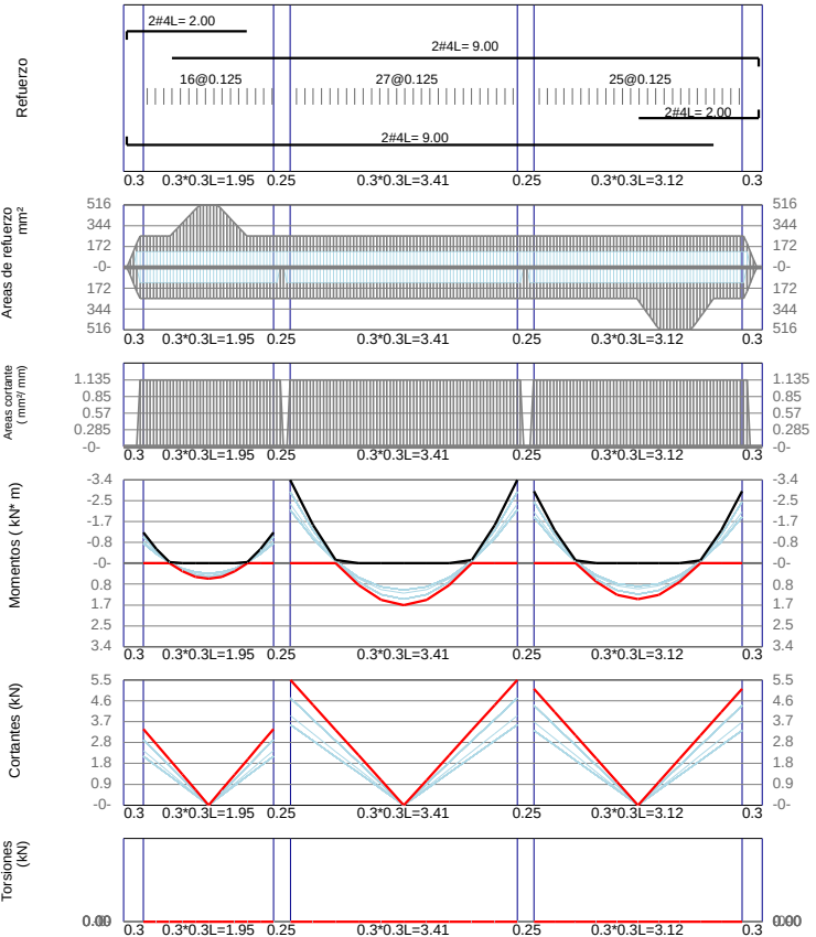
VCP5 / Base F'c=21\text{Mpa} Fy=420\text{Mpa} d'=60\text{mm}
