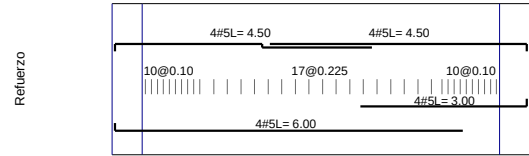
VP10 / Story2 F'c=21Mpa Fy=420Mpa d'=60mm
