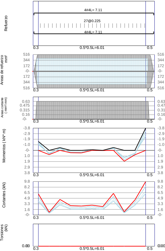
VCP7 / Base F´c=21Mpa Fy=420Mpa d'=60mm
