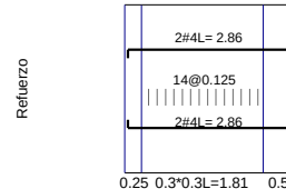
VCP4 / Base F´c=21Mpa Fy=420Mpa d'=60mm
