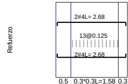
VCP3 / Base F´c=21Mpa Fy=420Mpa d'=60mm
