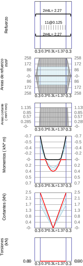
VCP9 / Base F´c=21Mpa Fy=420Mpa d'=60mm
