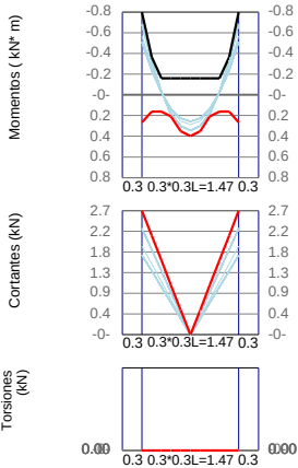
VCEI3(1) / Base F´c=21Mpa Fy=420Mpa d'=60mm
