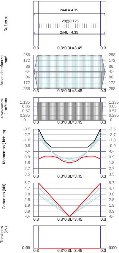
VCEI3(1) / Base F´c=21Mpa Fy=420Mpa d'=60mm
