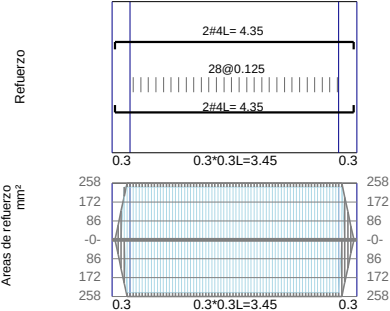
VCEI4(1) / Base F´c=21Mpa Fy=420Mpa d'=60mm
