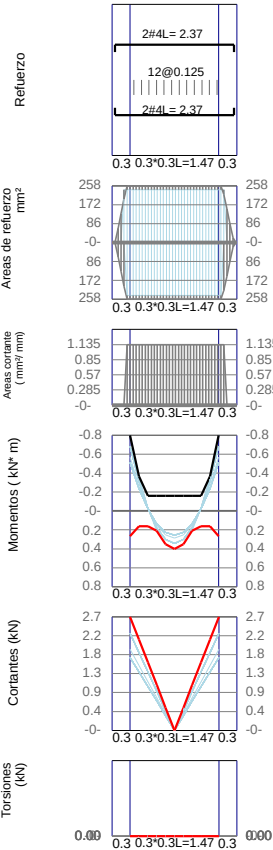
VCEI1(1) / Base F´c=21Mpa Fy=420Mpa d'=60mm
