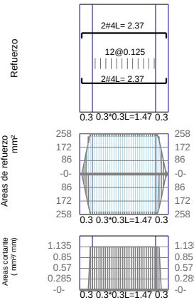
VCEI2(1) / Base F´c=21Mpa Fy=420Mpa d'=60mm
