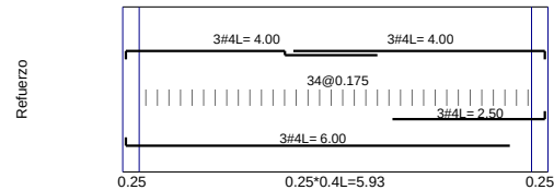
VCAnd4 / Base F´c=21Mpa Fy=420Mpa d'=60mm
