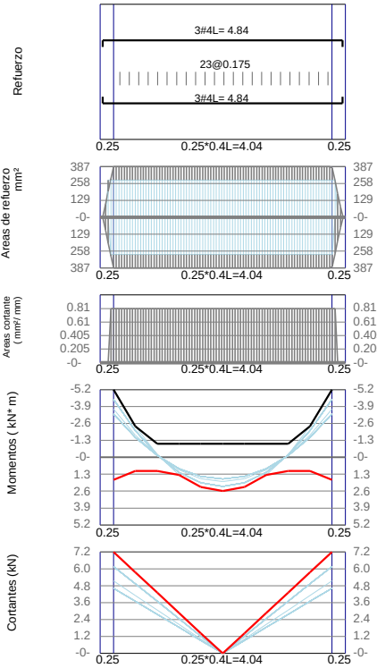
VCAnd2 / Base F'c=21Mpa Fy=420Mpa d'=60mm
