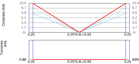
VCEI1(1) / Base F´c=21Mpa Fy=420Mpa d'=60mm
