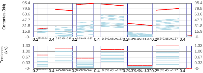
VB-4 / Story1 F'c=21Mpa Fy=420Mpa d'=60mm
