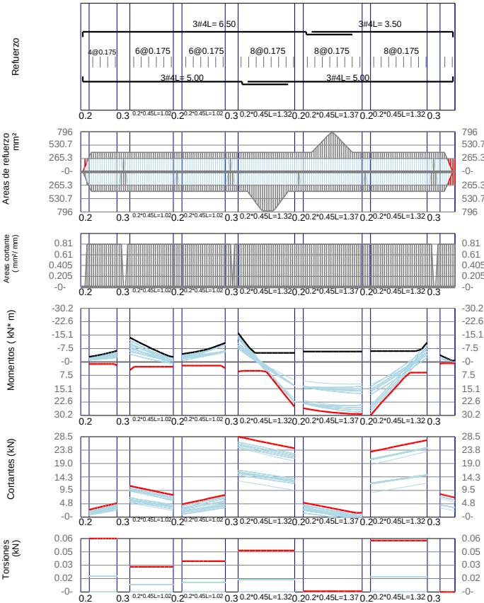
VB-2 / Story1 F'c=21Mpa Fy=420Mpa d'=60mm
