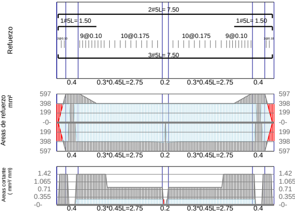
VB-5 / Story1 F'c=21Mpa Fy=420Mpa d'=60mm
