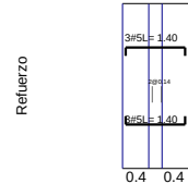
VCB-10 / Base F'c=21Mpa Fy=420Mpa d'=60mm
