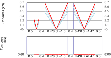
VCB-5 / Base F´c=21Mpa Fy=420Mpa d'=60mm
