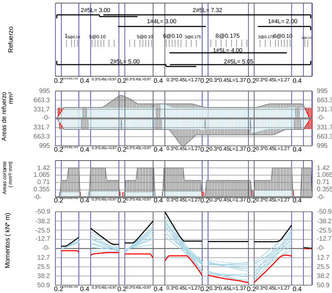
VB-3 / Story1 F'c=21Mpa Fy=420Mpa d'=60mm
