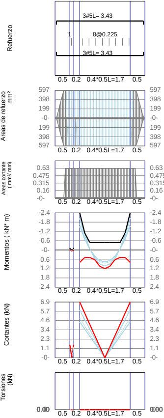
VCB-5 / Base F´c=21Mpa Fy=420Mpa d'=60mm
