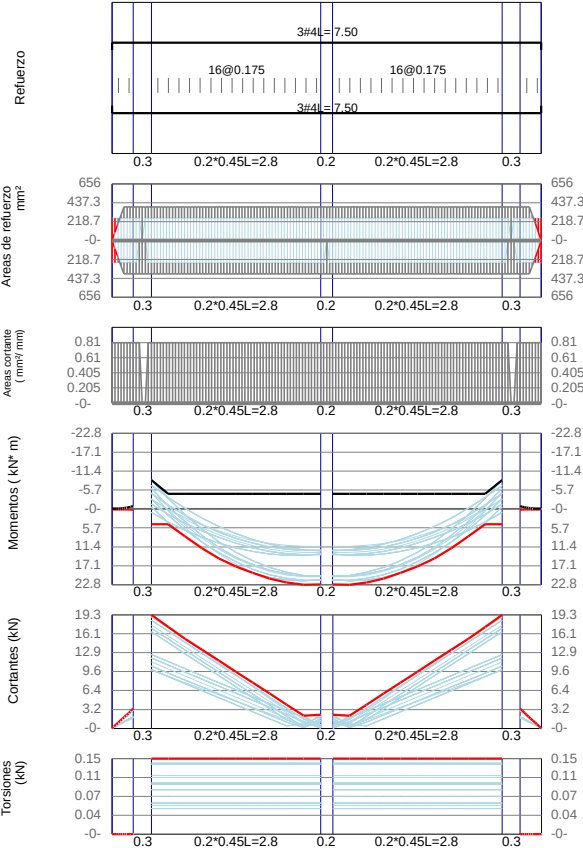
VB-4 / Story1 F'c=21Mpa Fy=420Mpa d'=60mm
