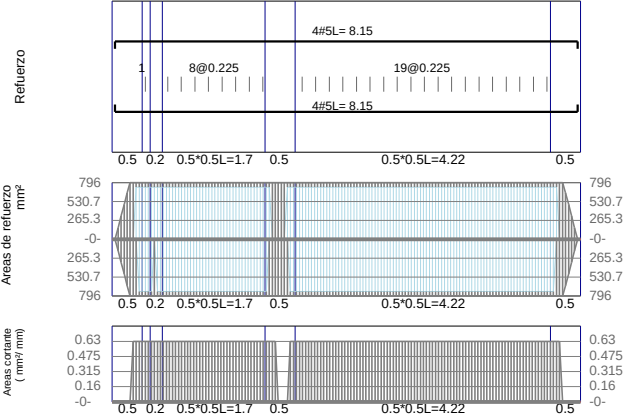
VCB-6 / Base F´c=21Mpa Fy=420Mpa d'=60mm
