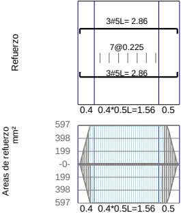
VC2-8 / Base F'c=21Mpa Fy=420Mpa d'=60mm
