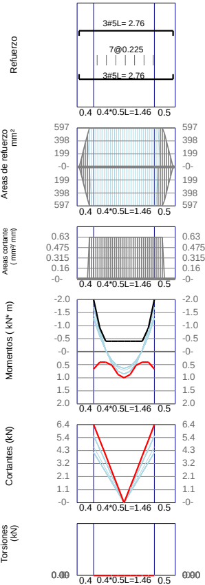
VC2-5 / Base F'_c=21\text{Mpa} F_y=420\text{Mpa} d'=60\text{mm}
