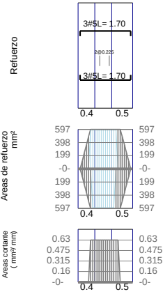
VC2-17 / Base F'c=21\text{Mpa} Fy=420\text{Mpa} d'=60\text{mm}
