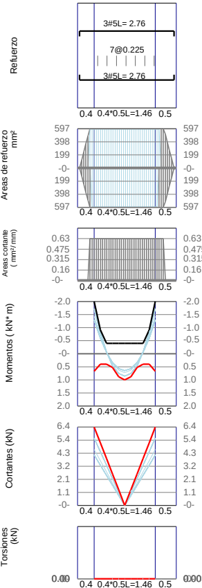
VC2-9 / Base F'c=21Mpa Fy=420Mpa d'=60mm
