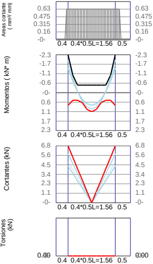
VC2-9 / Base F'c=21Mpa Fy=420Mpa d'=60mm
