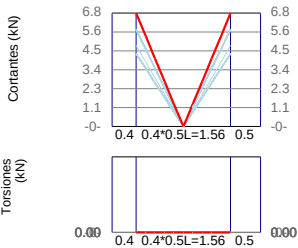
VC2-5 / Base F'_c=21\text{Mpa} F_y=420\text{Mpa} d'=60\text{mm}
