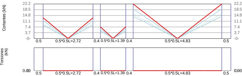
VC2-16 / Base F'c=21\text{Mpa} Fy=420\text{Mpa} d'=60\text{mm}
