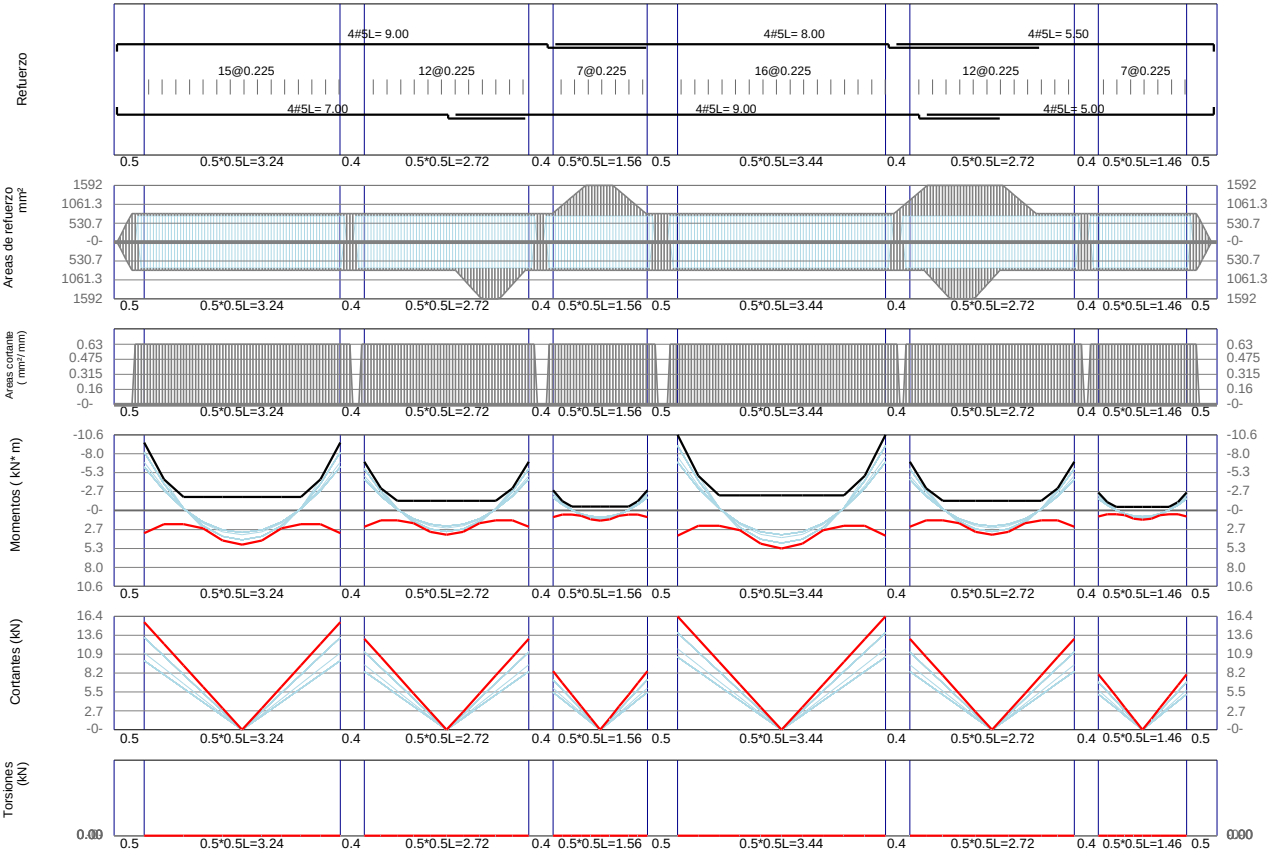
VC2-7 / Base F'c=21Mpa Fy=420Mpa d'=60mm
