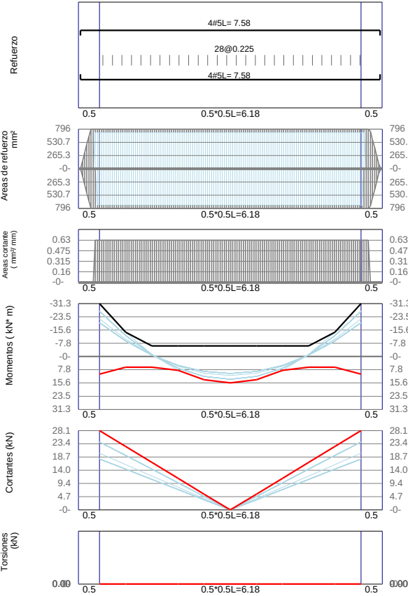
VC2-1 / Base F'c=21Mpa Fy=420Mpa d'=60mm
