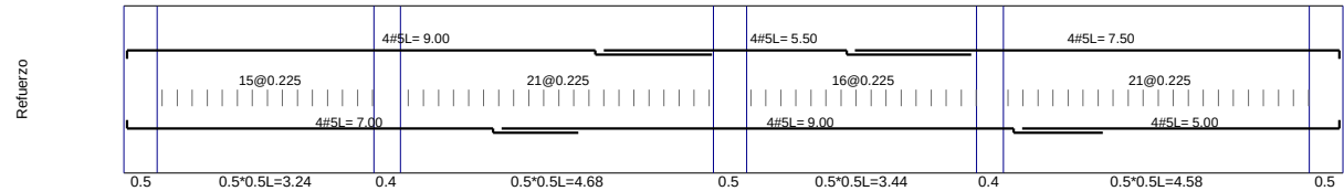
VC2-10 / Base F'c=21Mpa Fy=420Mpa d'=60mm
