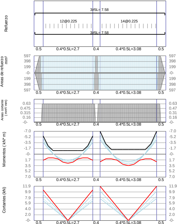
VC2-2 / Base F'c=21Mpa Fy=420Mpa d'=60mm
