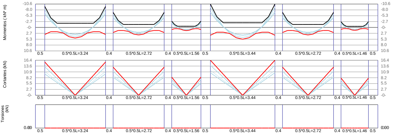
VC2-7 / Base F'c=21Mpa Fy=420Mpa d'=60mm
