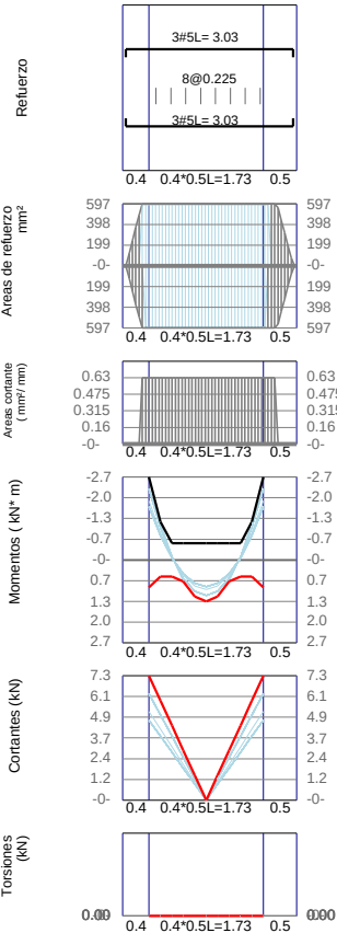
VCSec-4 / Base F´c=21Mpa Fy=420Mpa d'=60mm
