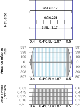
VCSec-7 / Base F´c=21Mpa Fy=420Mpa d'=60mm
