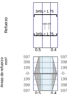
VCSec-10 / Base F'c=21\text{Mpa} Fy=420\text{Mpa} d'=60\text{mm}
