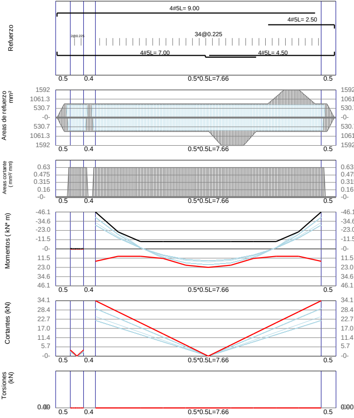
VCSec-14 / Base F'_c=21\text{Mpa} F_y=420\text{Mpa} d'=60\text{mm}
