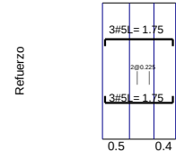
VCSec-12 / Base F'_c=21\text{Mpa} F_y=420\text{Mpa} d'=60\text{mm}
