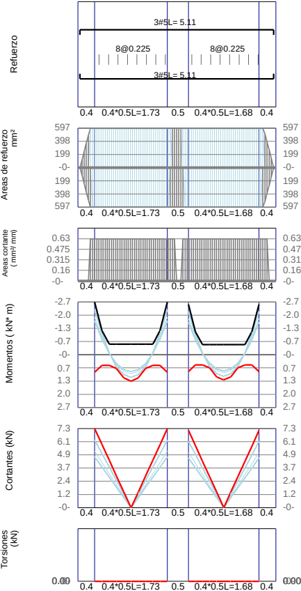
VCSec-6 / Base F´c=21Mpa Fy=420Mpa d'=60mm
