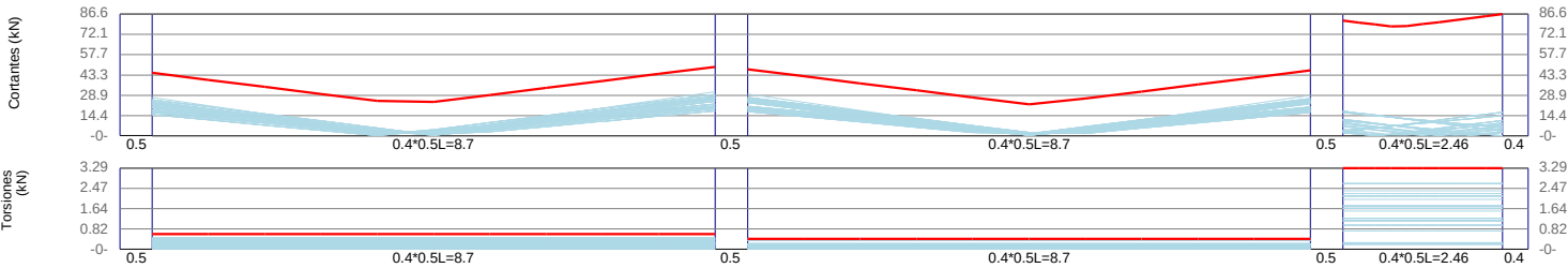
VBb18 / Story3 F'c=21Mpa Fy=420Mpa d'=60mm
