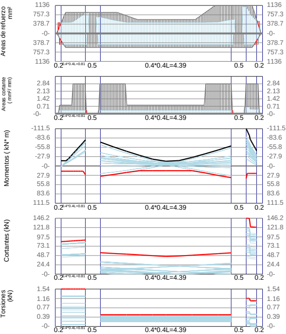
VBb14 / Story2 F'c=21Mpa Fy=420Mpa d'=60mm
