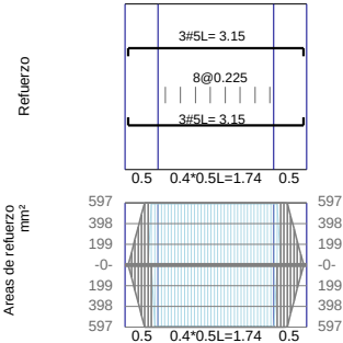
VCBb11 / Base F'c=21Mpa Fy=420Mpa d'=60mm
