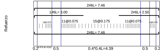
VBB13 / Story2 F'c=21Mpa Fy=420Mpa d'=60mm
