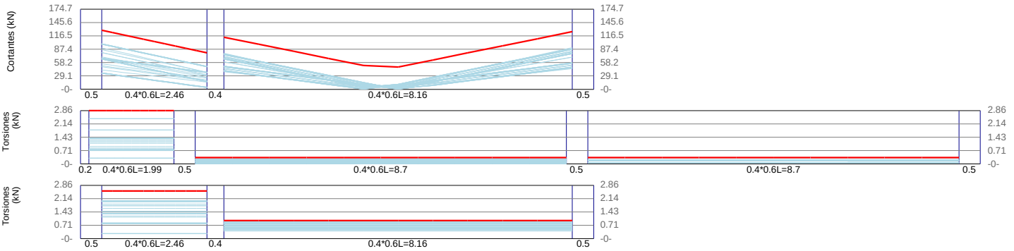
VBb8 / Story2 F'c=21Mpa Fy=420Mpa d'=60mm
