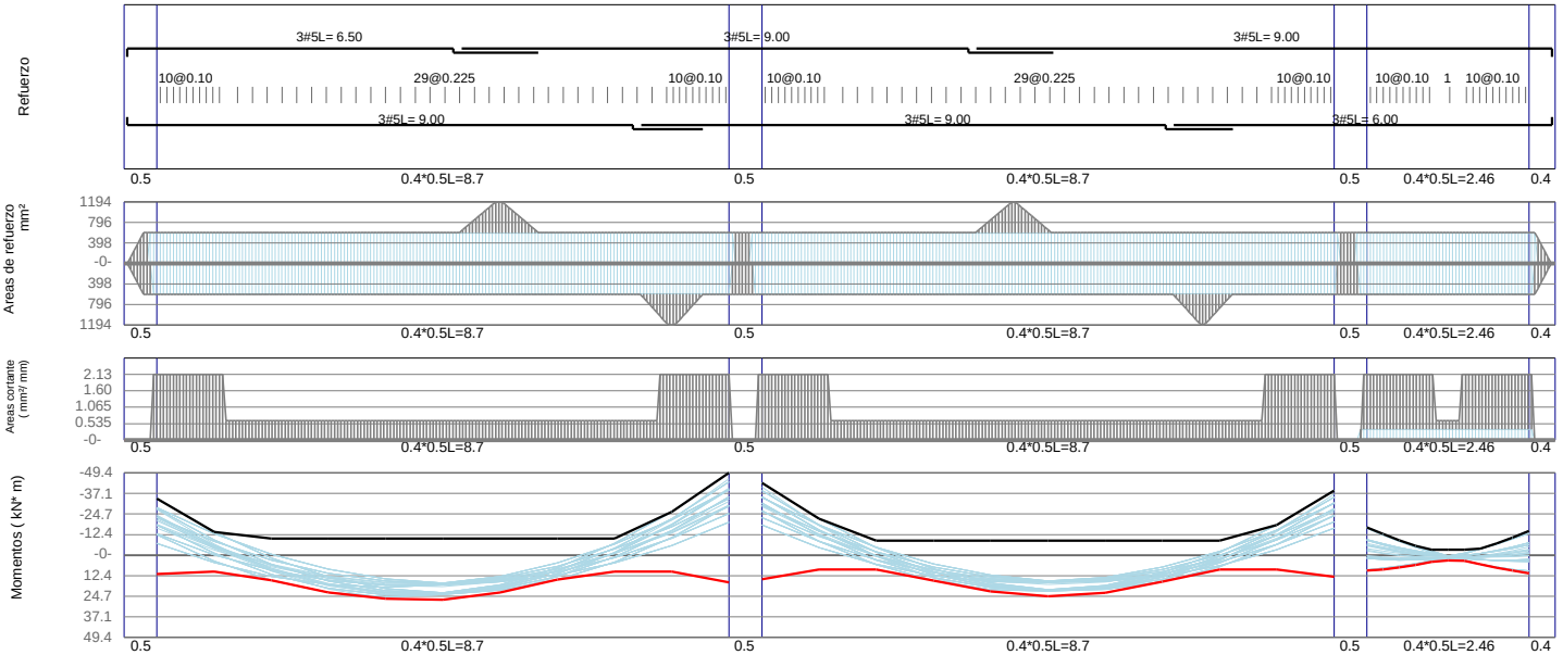
VBb17 / Story3 F'c=21Mpa Fy=420Mpa d'=60mm
