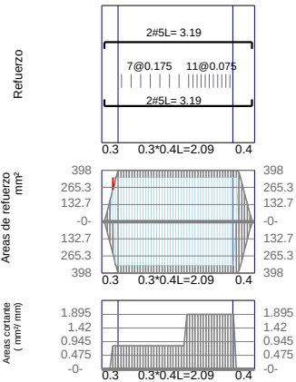
VBb19 / Story3 F'c=21Mpa Fy=420Mpa d'=60mm
