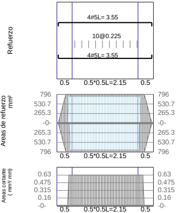
VCBb9 / Base F'c=21Mpa Fy=420Mpa d'=60mm
