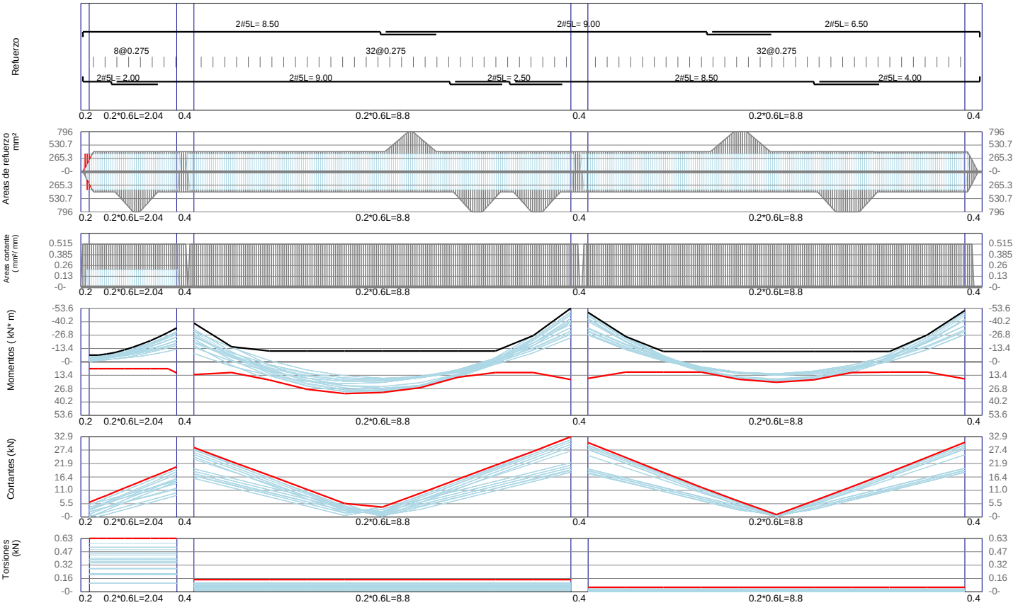
VBbR1 / Story2 F'c=21Mpa Fy=420Mpa d'=60mm
