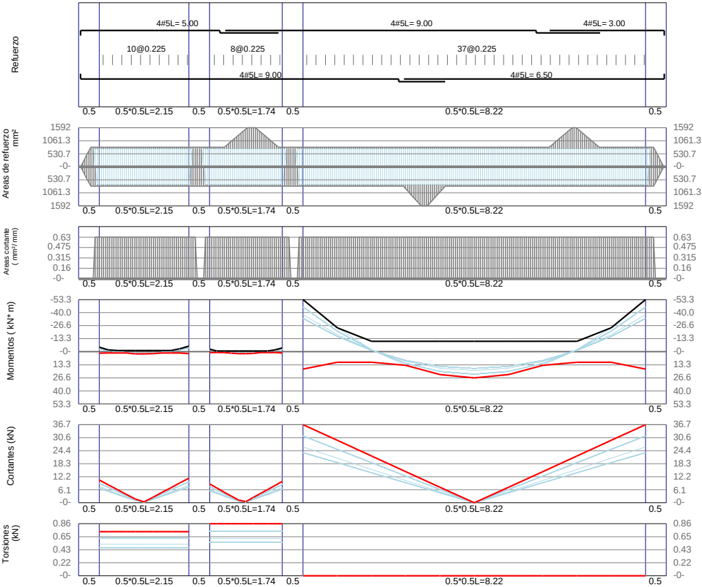
VCBb11 / Base F'c=21Mpa Fy=420Mpa d'=60mm
