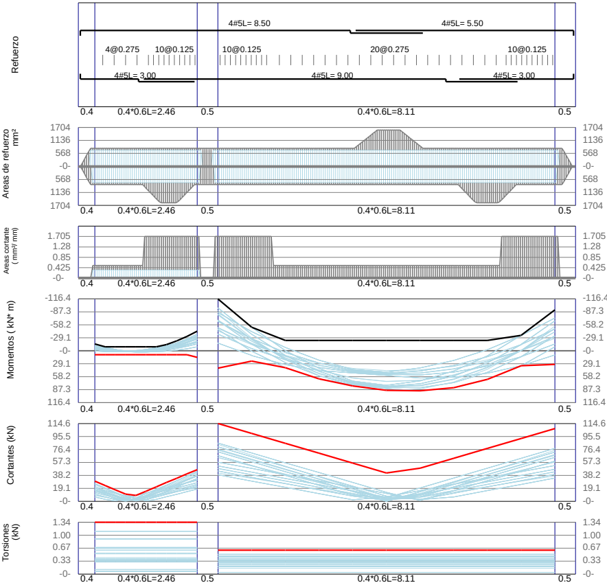
VBb8 / Story2 F'c=21Mpa Fy=420Mpa d'=60mm
