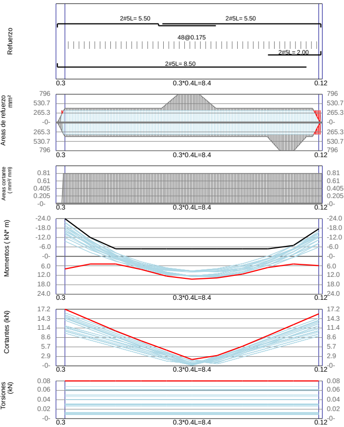
VBb18 / Story3 F'c=21Mpa Fy=420Mpa d'=60mm
