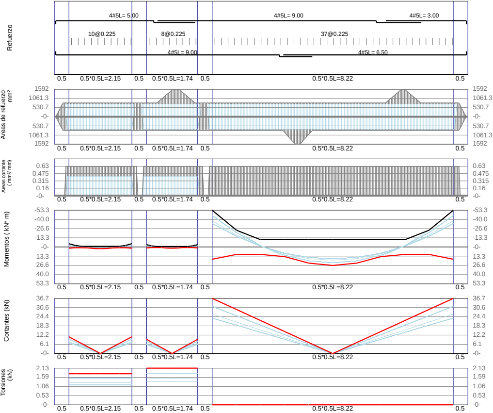
VCBb9 / Base F'c=21Mpa Fy=420Mpa d'=60mm
