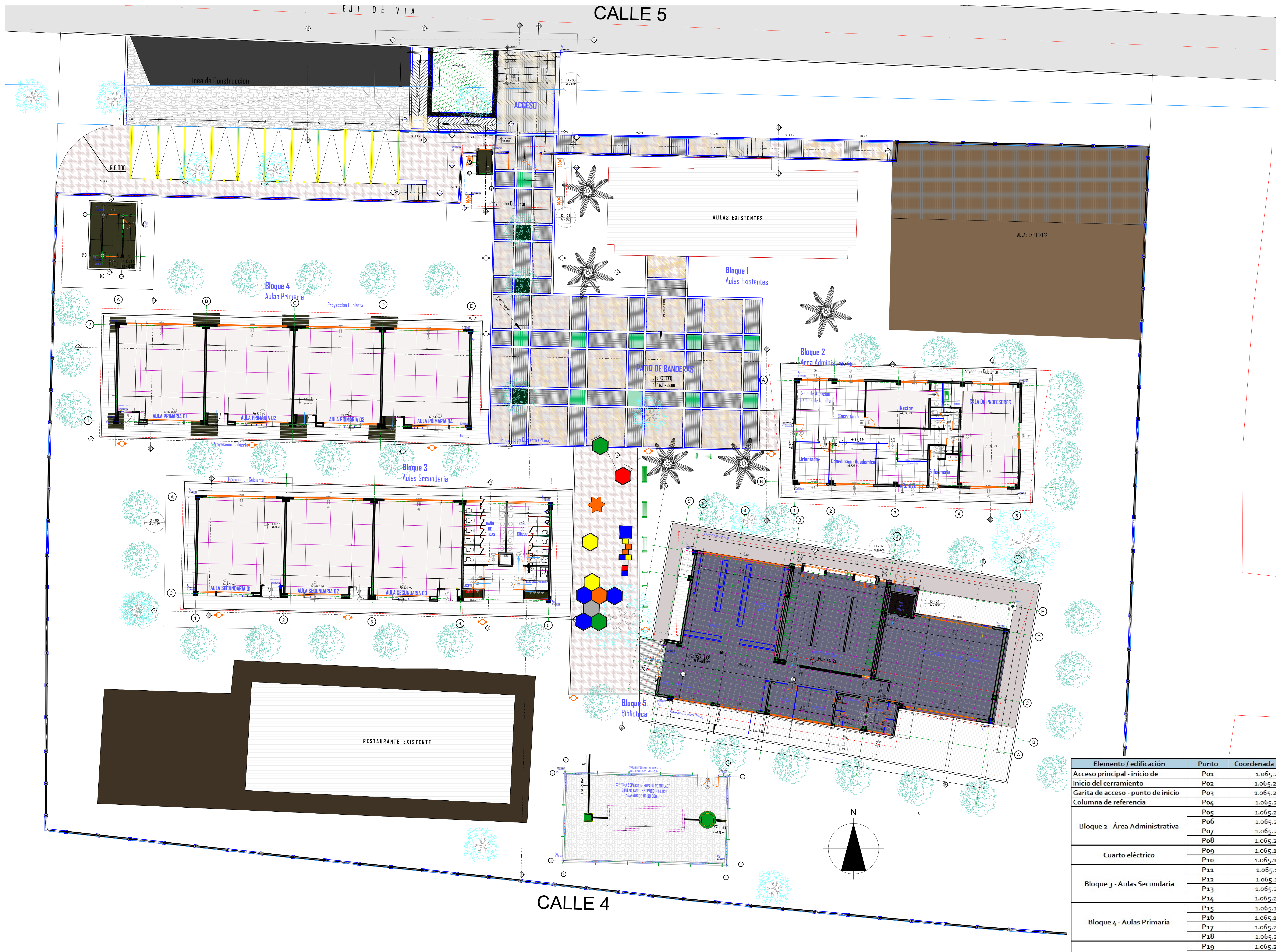
Planta de Trazado y Replanteo 1:150
