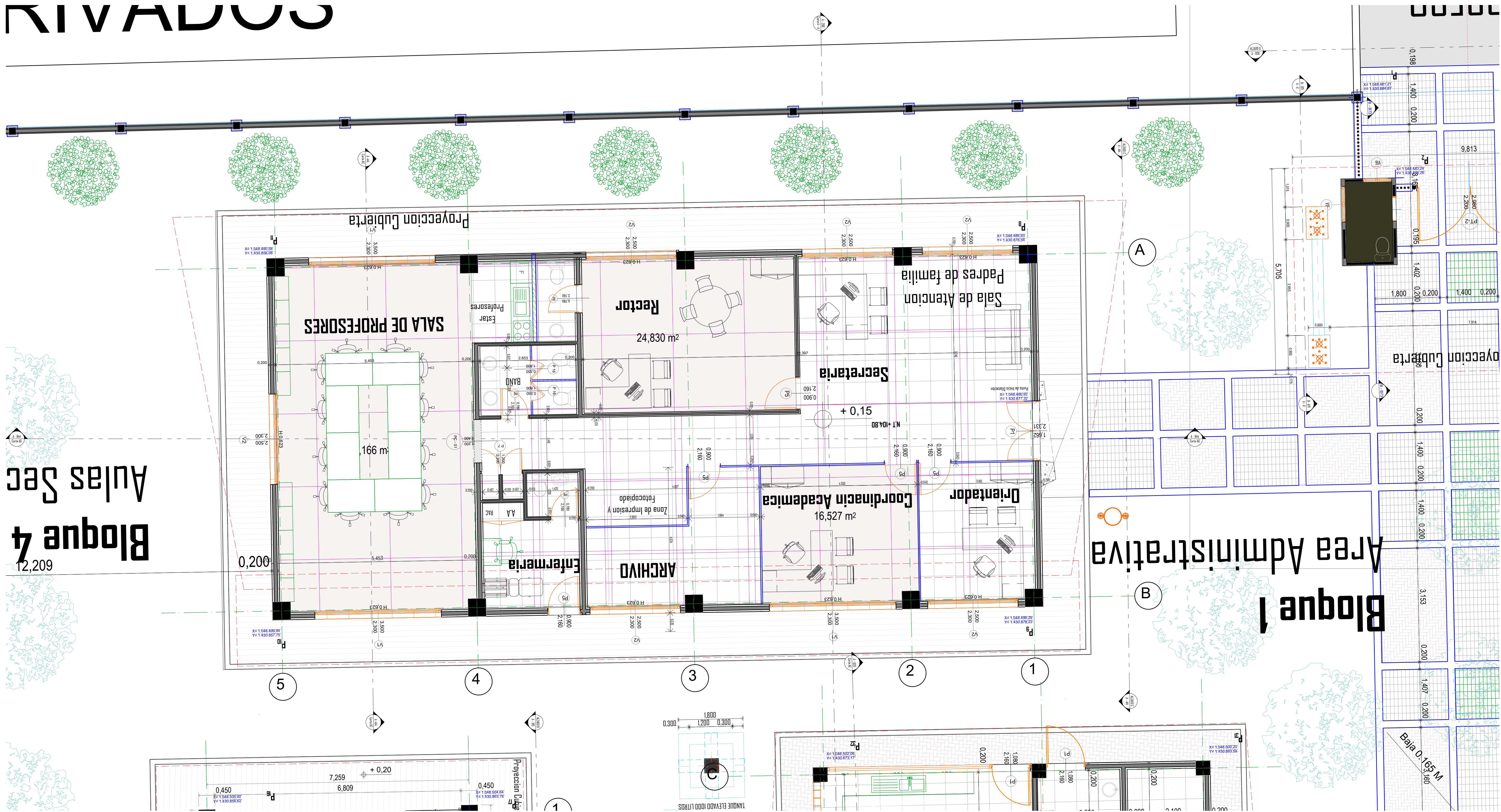
1 Planta Arquitectonica Bloque Administrativo 1:50
