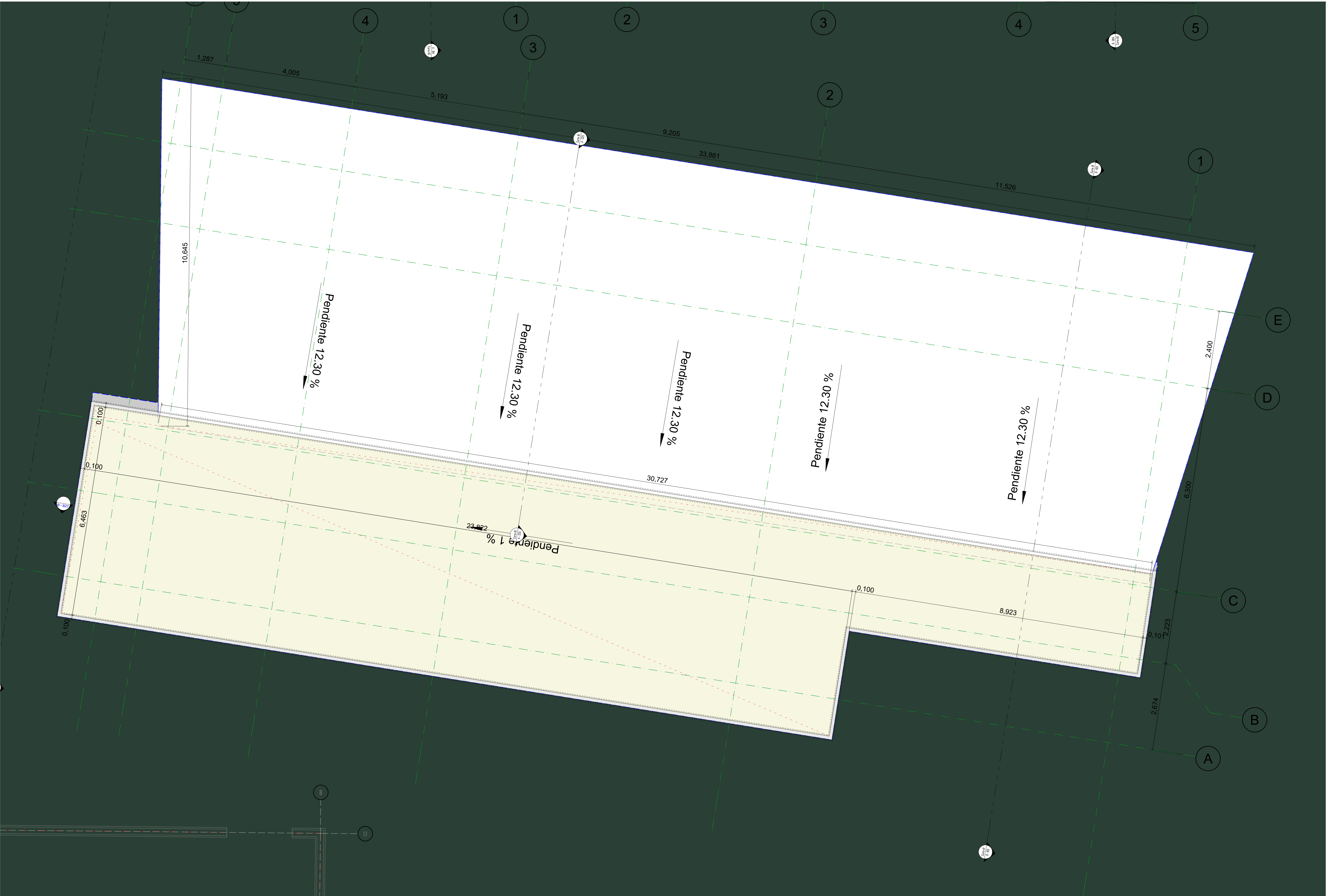
Planta Cubierta Biblioteca 1:50
