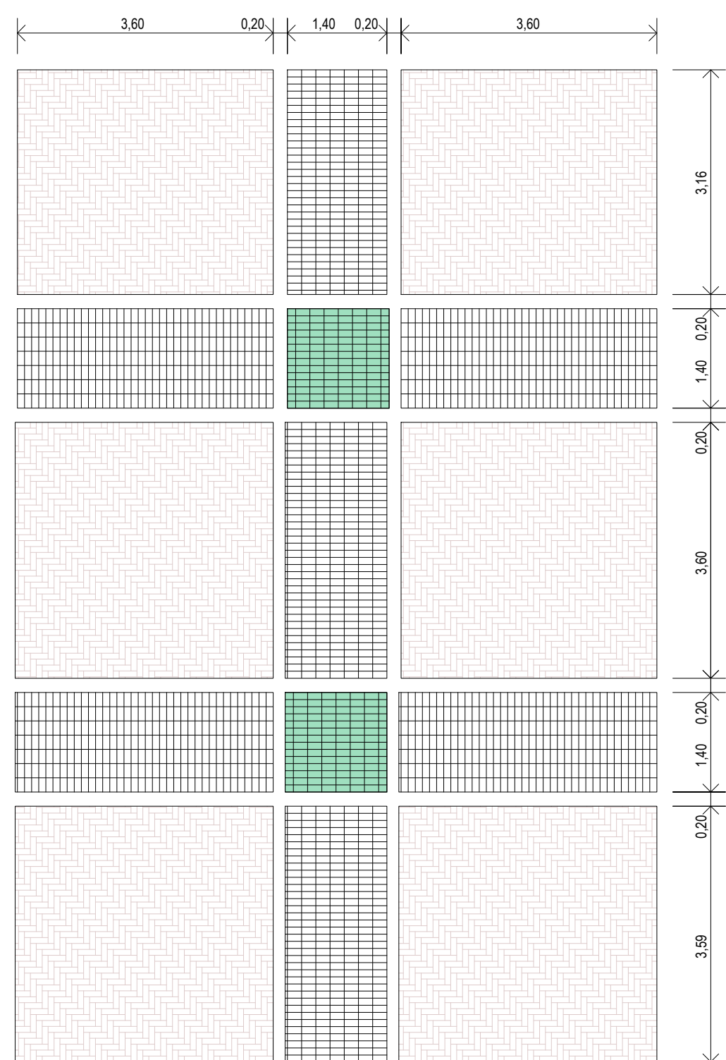
D-03 DETALLE PLANTA DE PATIO BANDERAS 1:75
