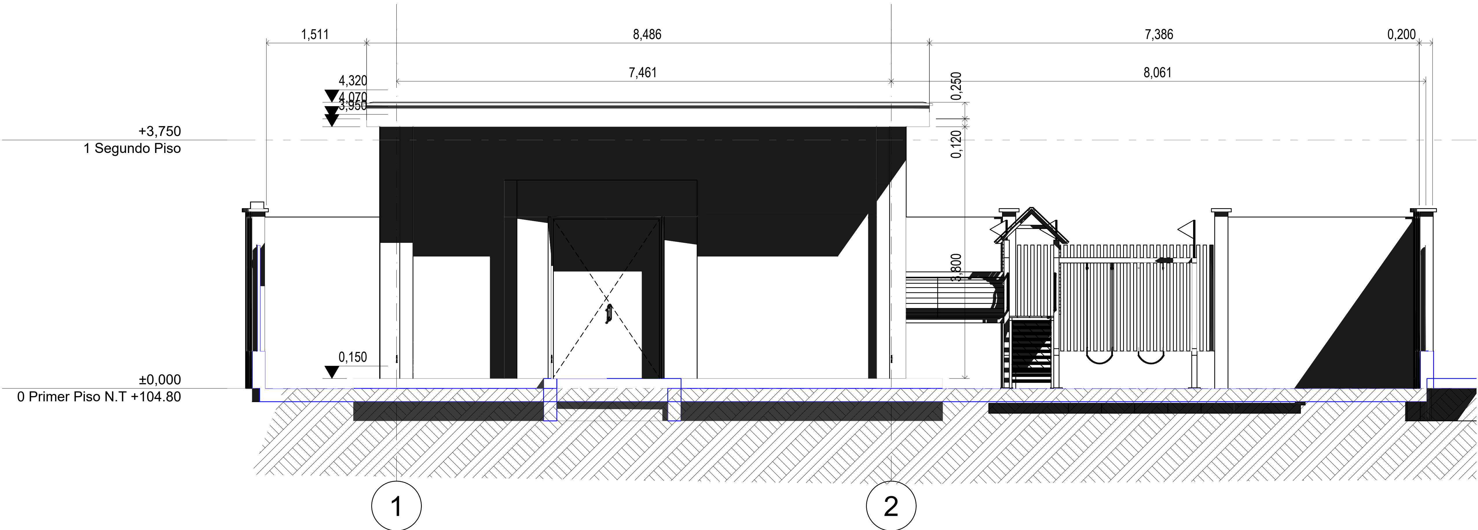
Alzado Aula Prescolar 1:33
