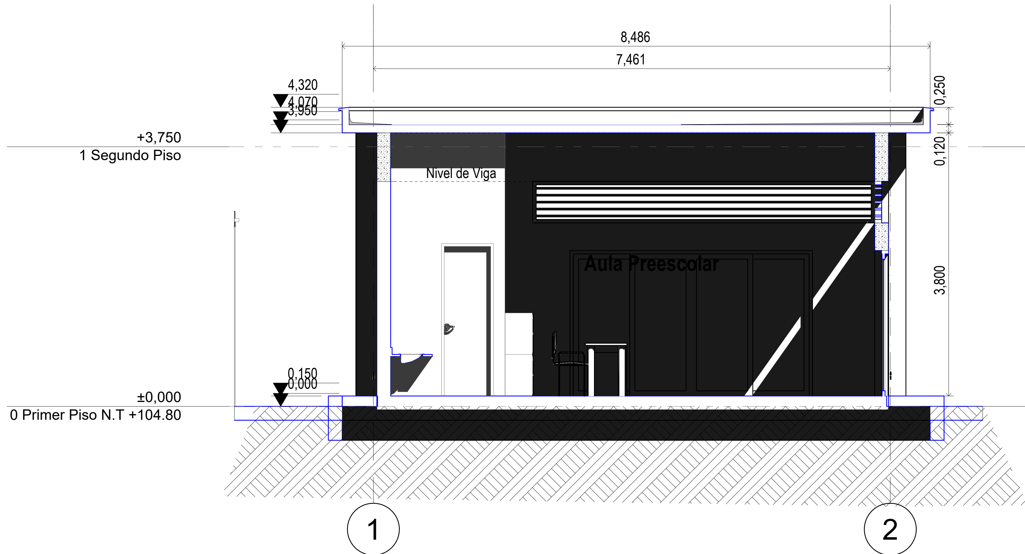
Corte Aula Prescolar 1:33
