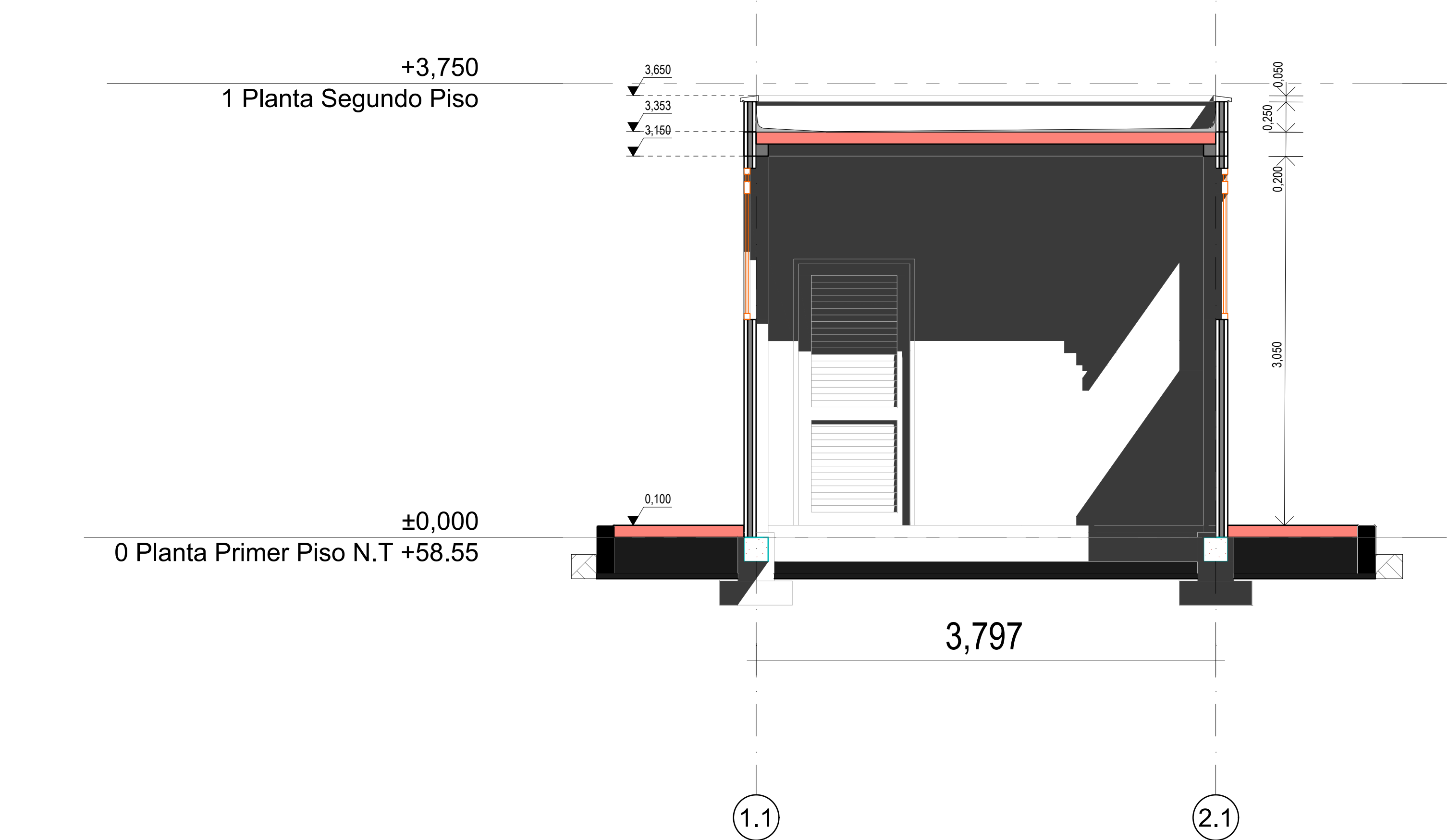
Corte Cuarto Elctrico B 08 1:30
