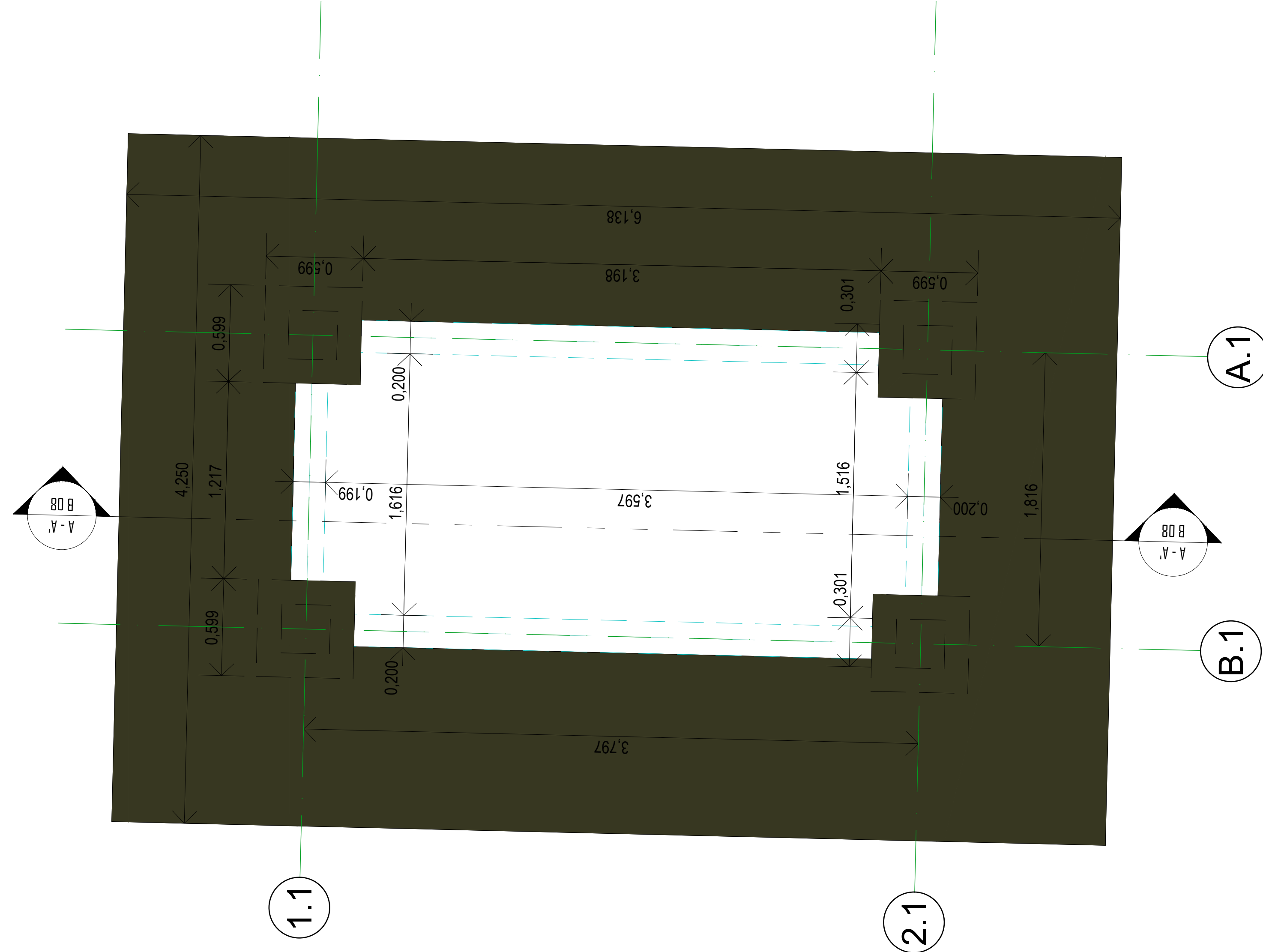
Cuarto Elctrico Cimentacion 1:20
