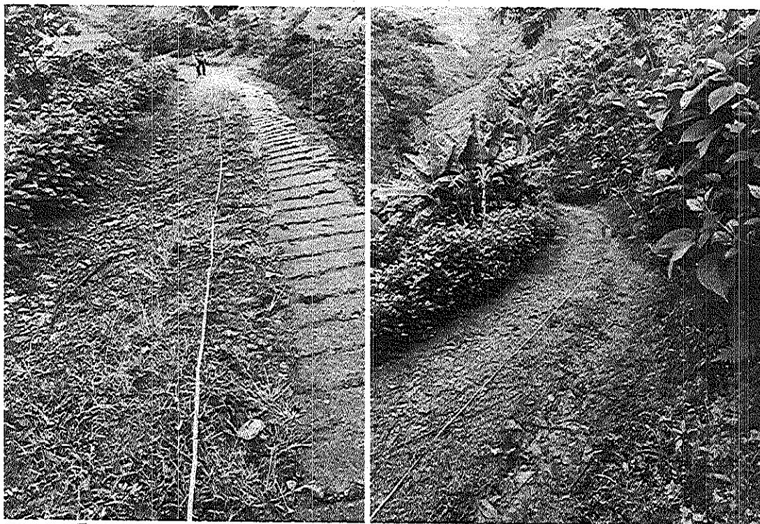
Figura 2. Evidencias fotográficas estado del tramo para construcción de placa huella.
