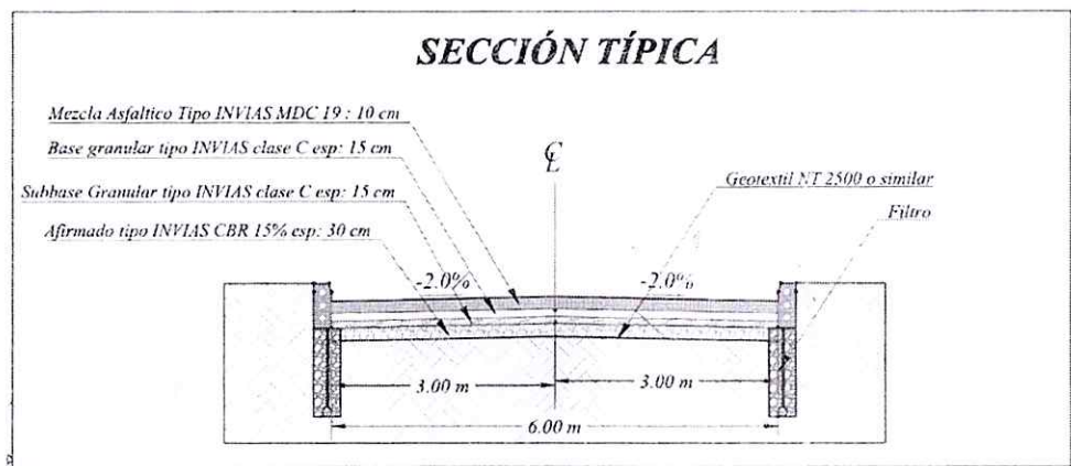
Figura 2. Sección típica propuesta para el corredor vial a intervenir.
