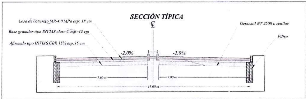
Figura 3. Sección Típica propuesta para el corredor vial a intervenir.
