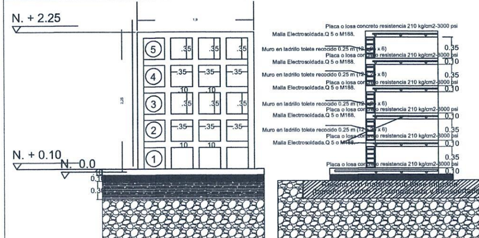
FACHADA LATERAL
