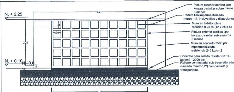
FACHADA FRONTAL
