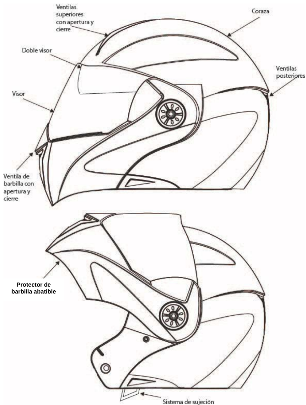
Figura ilustrativa 2. Casco de Seguridad para Motociclista Tipo "2" Abatible o Escualizable
