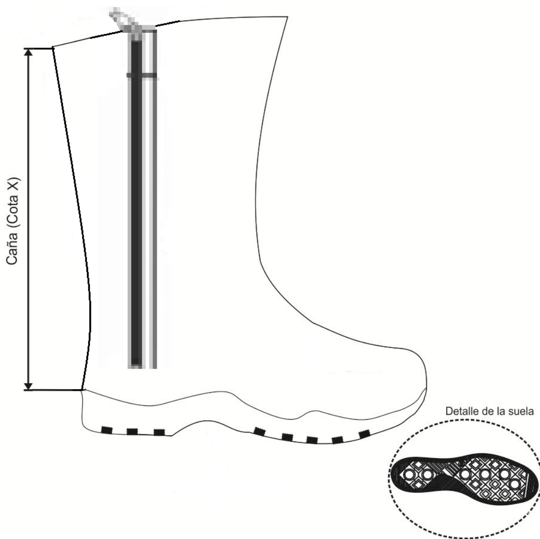
Figura 8. Vista ilustrativa diseño del Zapatón con cierre de cremallera
