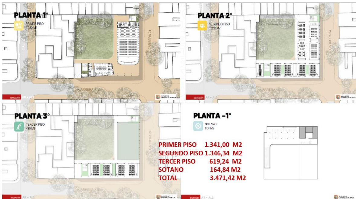
Figura 6. Vistas en planta proyecto Institución Educativa Oficial República de Argentina sede Principal.
