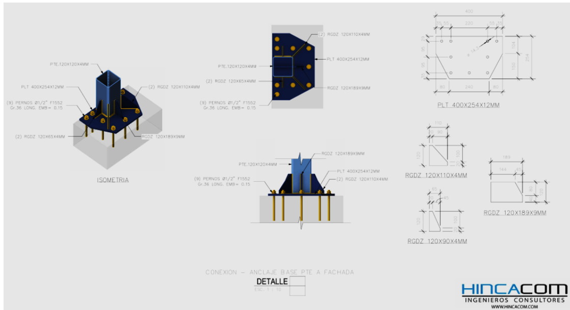
Figura 24. Detallado de placa base marco metálico
