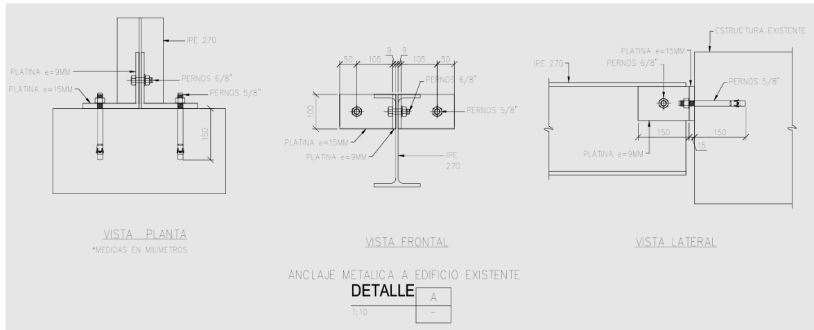
Figura 20. Detalle A — conexión de la estructura metálica nueva con la fachada existente (vista en planta, frontal y lateral). Fuente: planos estructurales, procedimiento Ing. Estructural Andrés Hincapié.
