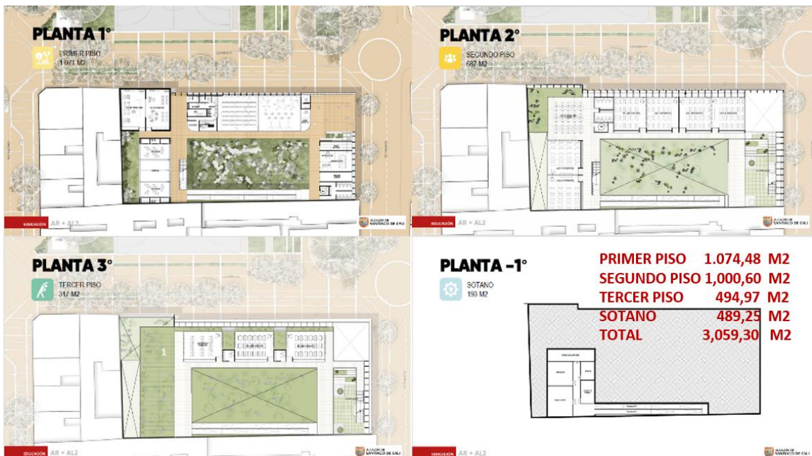
Figura 9. Vistas en planta proyecto Institución Educativa Oficial República de Argentina sede Policarpa Salavarría.
