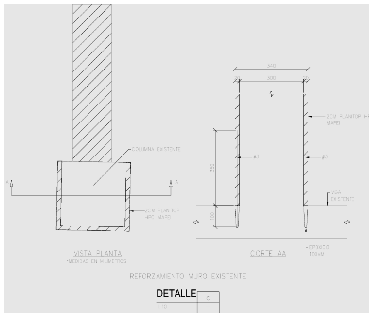
Figura 21. Detalle de reforzamiento de columnas de fachada con Planitop HPC — vista en planta y corte AA. Fuente: planos estructurales, procedimiento Ing. Estructural Andrés Hincapié.
