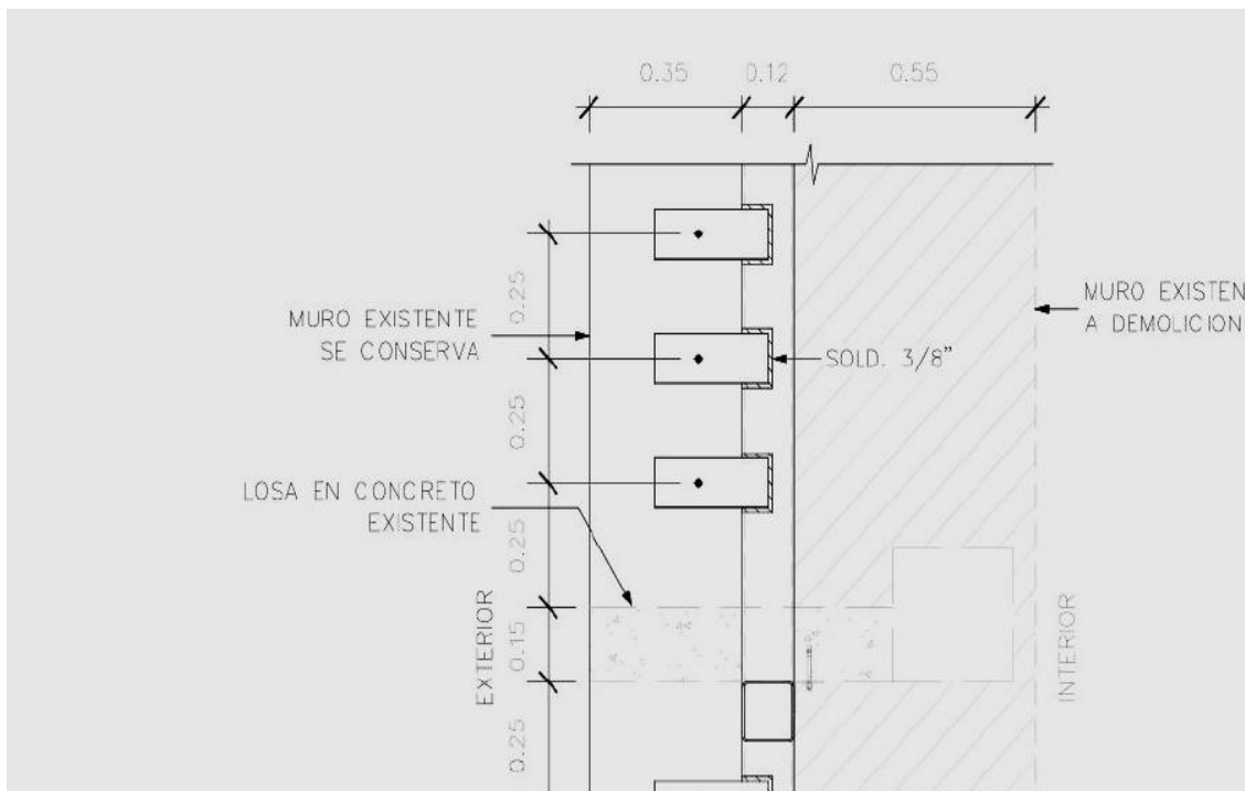
Figura 23. Detalle de amarre lateral del marco metálico al concreto existente (Detalle F). Fuente: planos estructurales.
