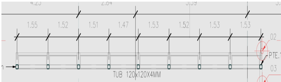
Figura 22. Marco metálico de reforzamiento de fachada entre ejes A y C — tubular 120x120x4mm. Fuente: planos estructurales.
