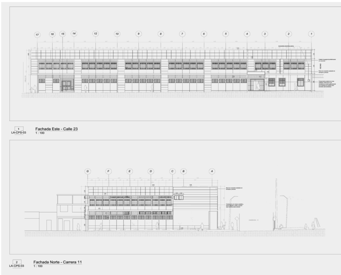
Figura 15. Levantamiento arquitectónico existente - alzados este (calle 23) y norte (carrera 11).
