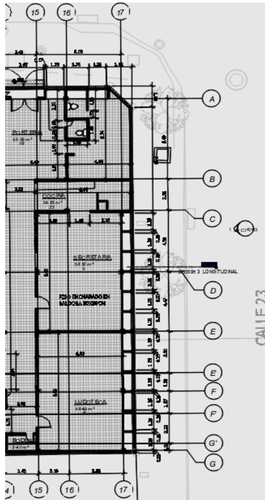
Figura 19. Conservar pórticos de concreto eje 15 y 17
