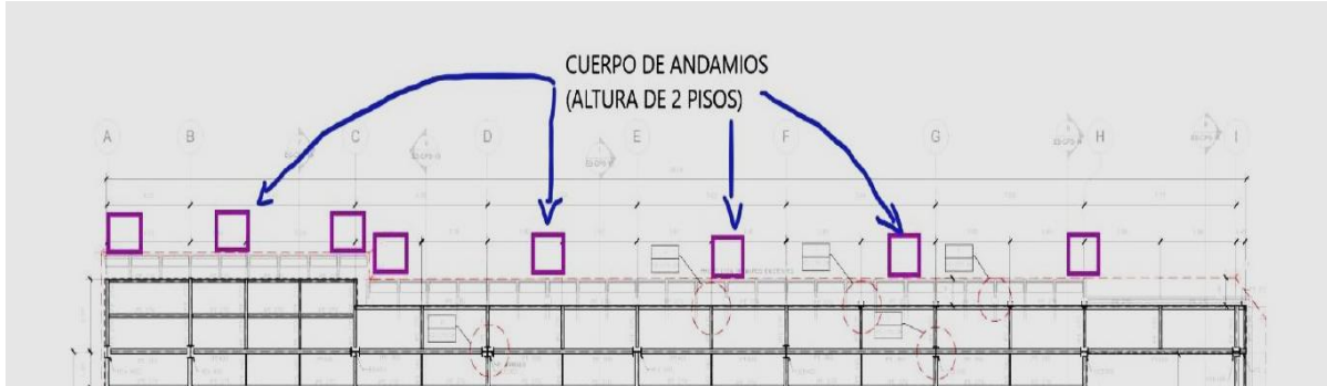
Figura 16. Esquema de localización de cuerpos de andamios sobre la Carrera 11, según posición de columnas existentes. Fuente: procedimiento Ing. Estructural Andrés Hincapié
