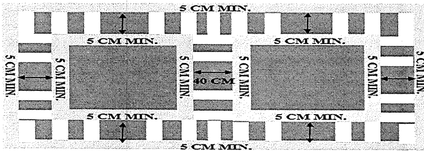
Imagen 1 (modelo de puestos de trabajo y libre circulación del técnico u operario (mecánico) con sus equipos y herramientas)
