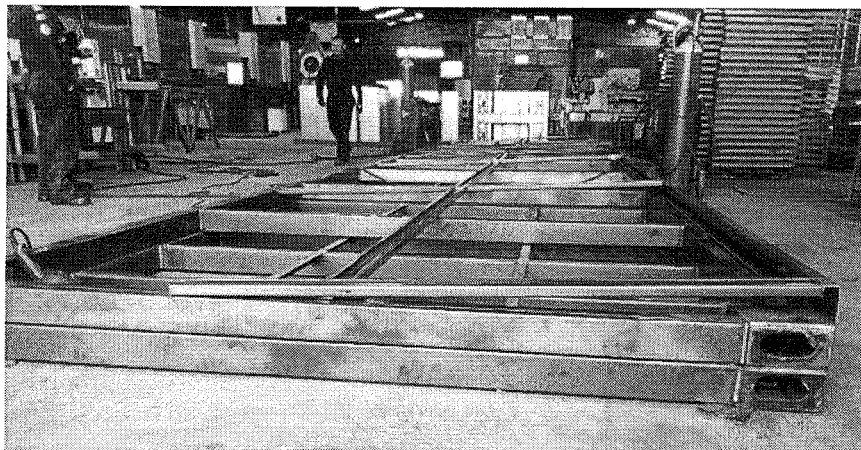
Foto 2 Base piso, base techo y caída
