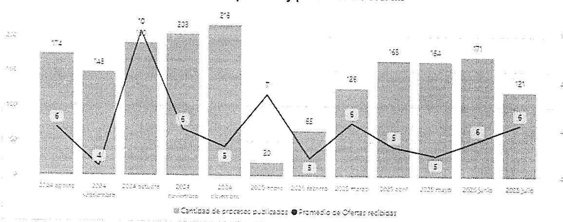
Cantidad de procesos y promedio de ofertas
