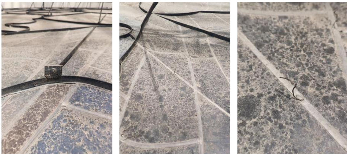
Figura 3. Vista de los detalles de: uniones de los marcos, empujados, enmasillado, y amarres sueltos por la pérdida de las varillas de refuerzo.
