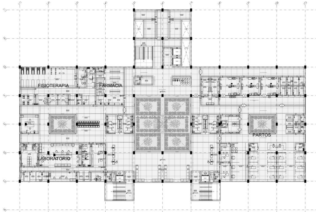
PLANTA ARQUITECTÓNICA PISO 2 (tomado de la planimetría del proyecto / Nombre archivo: UMA_IBG_TOL-A102_SEGUNDO_PISO_LABORATORIO_CLINICO_FISIOTERAPIA_FARMACIA_PARTOS.pdf)
