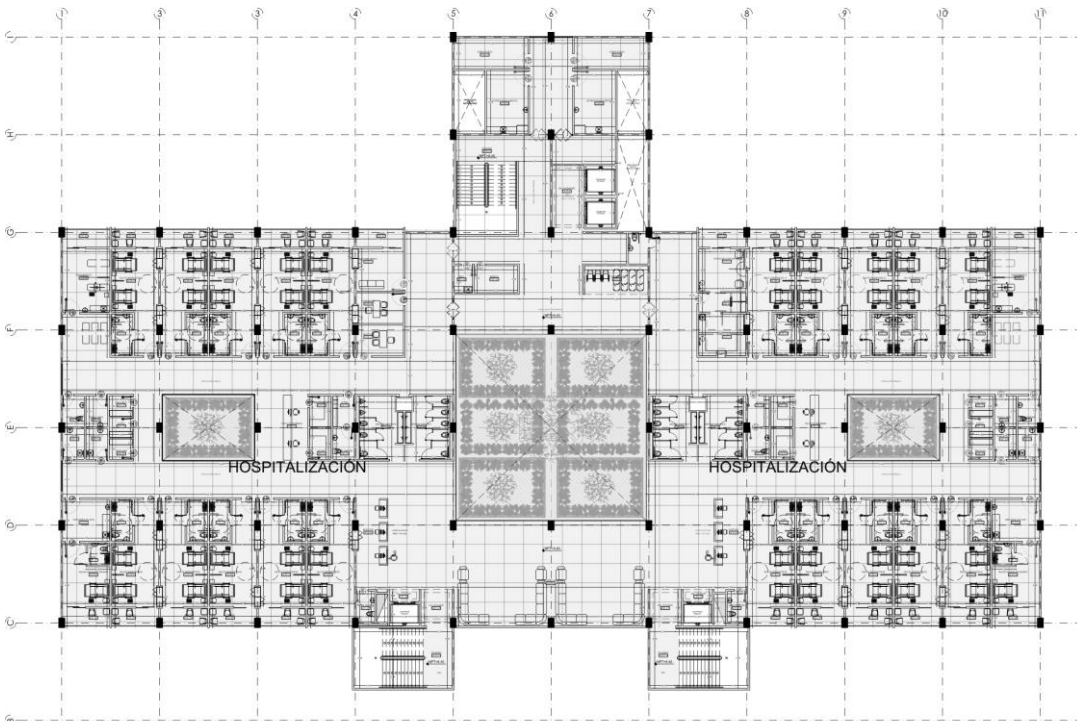
PLANTA ARQUITECTÓNICA PISO 3 (tomado de la planimetría del proyecto / Nombre archivo: UMA_IBG_TOL-A103_TERCER_PISO_HOSPITALIZACION.pdf)
