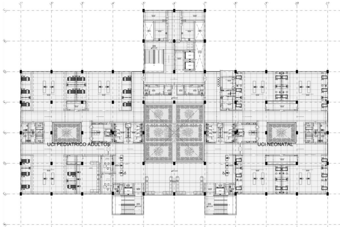
PLANTA ARQUITECTÓNICA PISO 4 (tomado de la planimetría del proyecto / Nombre archivo: UMA_IBG_TOL-A104_CUARTO_PISO_UCI.pdf)
