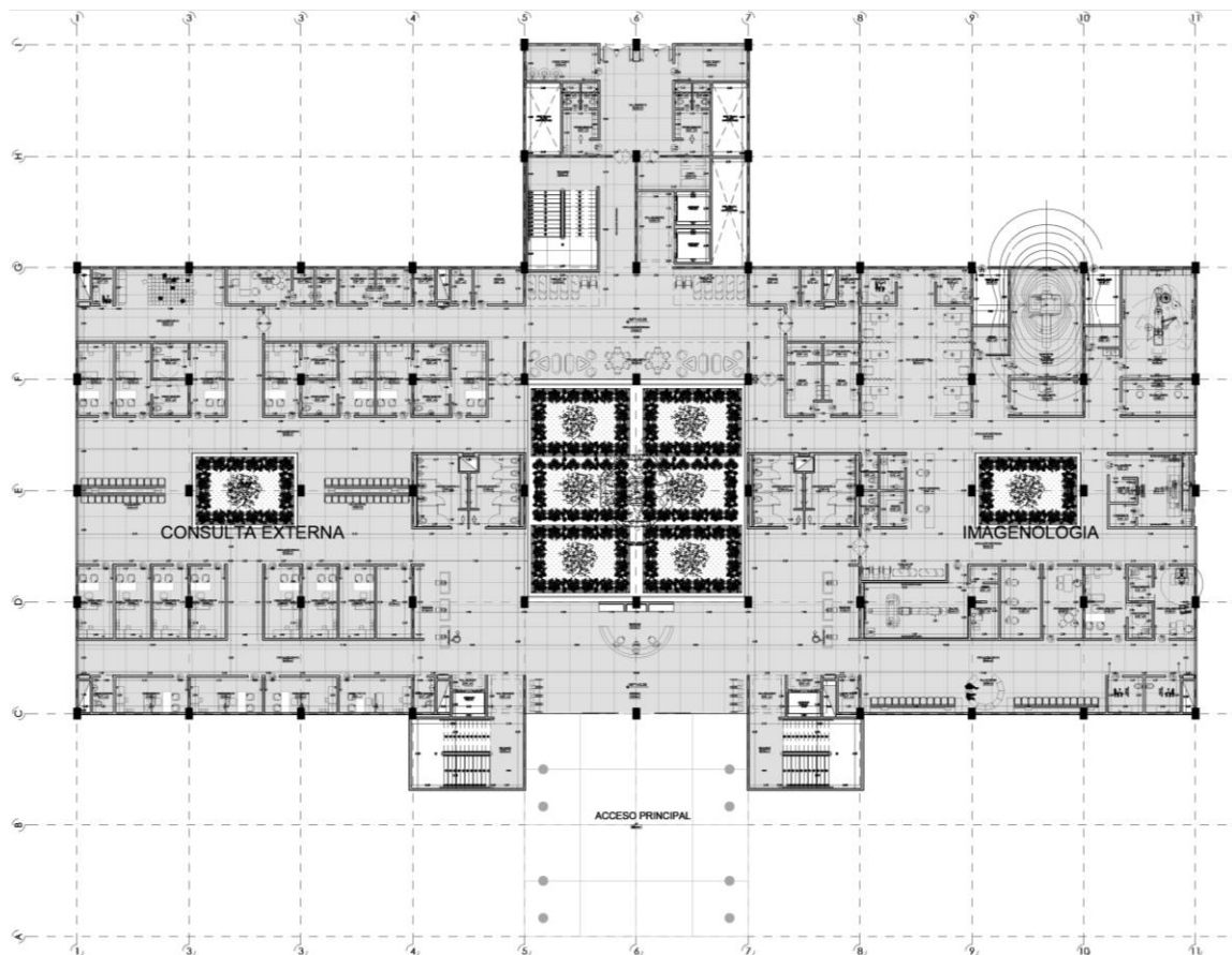
PLANTA ARQUITECTÓNICA PISO 1 (tomado de la planimetría del proyecto / Nombre archivo: UMA_IBG_TOL-A101_PRIMER_PISO_CONSULTA_EXTERNA_IMAGENOLOGIA.pdf)
