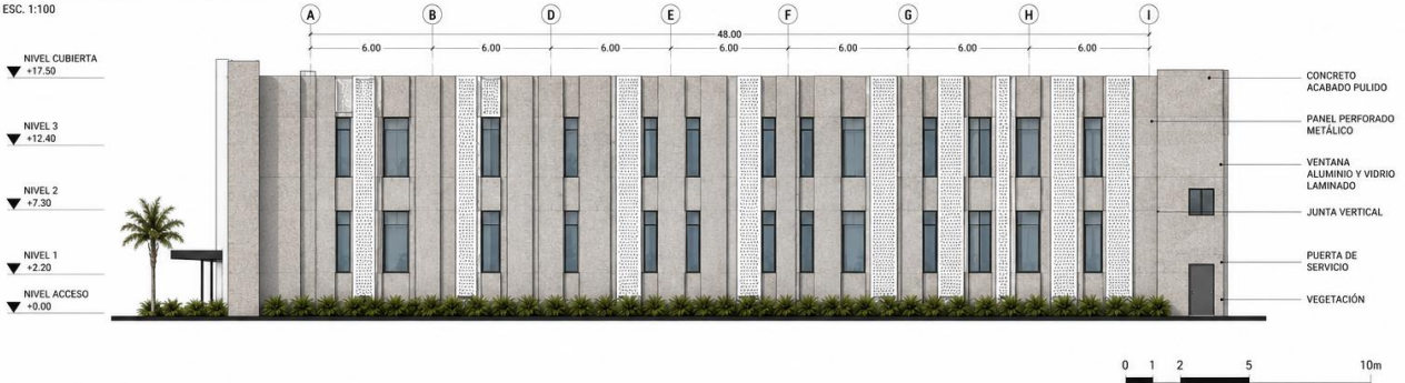
FACHADAS ARQUITECTÓNICAS (tomado de la planimetría del proyecto / Nombre archivo: FACHADAS.png )
