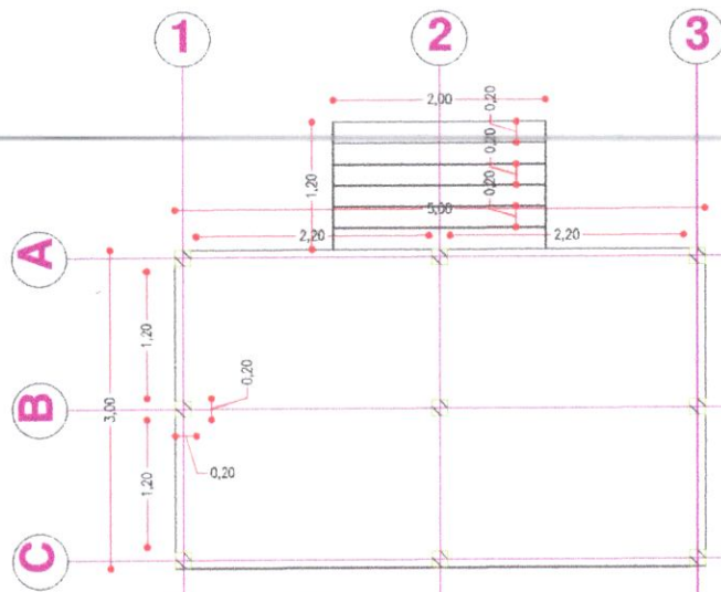
PLANTA ARQUITECTONICA
