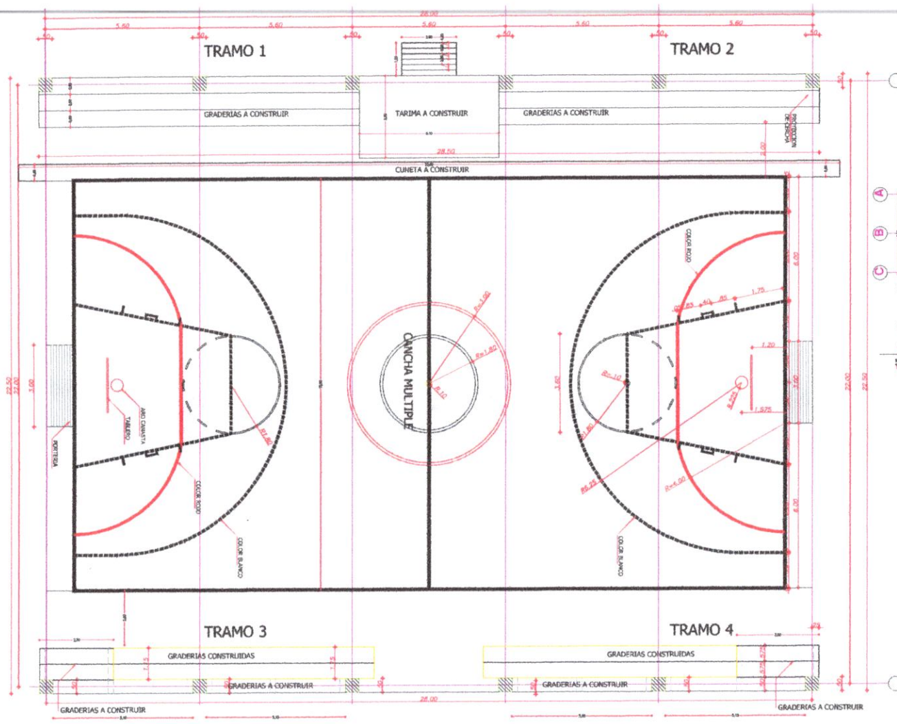
CONSTRUCCION DE TARIMA EN CONCRETO
