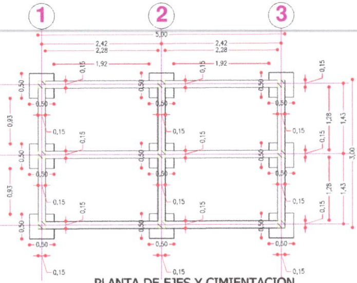
PLANTA DE EJES Y CIMIENTACION
