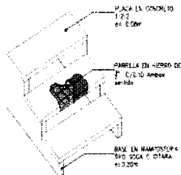
DETALLE ISOMETRICO
