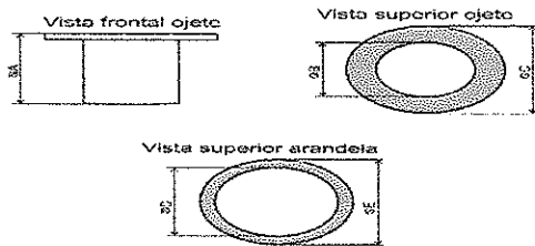
Figura 6. Vista ilustrativa de las medidas del ojete y la arandela
