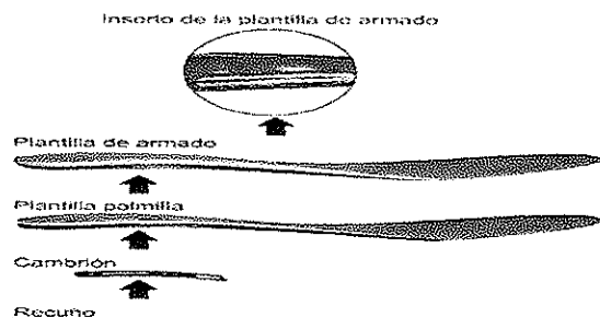
Figura 10 Vista ilustrativa del despliegue de plantilla de armado.
