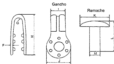
Figura 7. Vista ilustrativa de las medidas del gancho de extracción rápida
