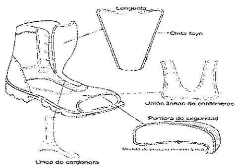
Figura 3. Despiece de la bota de seguridad
