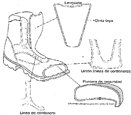
Figura 3. Despiece de la bota de seguridad
