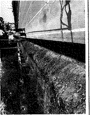
Suministro, extendida y compactación mecánica hasta densidad del 95% material de mejoramiento Recebo.
