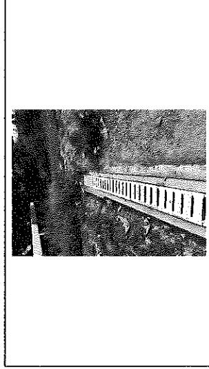
Instalación rejilla para cárcamo exterior de la pista con ancho 0,30 m. prefabricada en concreto reforzado. E= 0,06 m.
