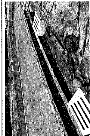
Suministro de rejilla para cárcamo interno de la pista con ancho 0,50 m. prefabricada en concreto reforzado. E= 0,06 m.
