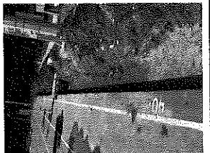
Suministro, extendida y compactación mecánica hasta densidad del 95% material de mejoramiento Recebo.
