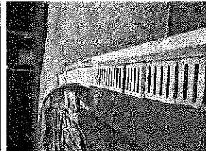
Instalación rejilla para cárcamo interno de la pista con ancho 0,50 m. prefabricada en concreto reforzado. E= 0,06 m. En la zona Suroccidente de la pista de atletismo.
