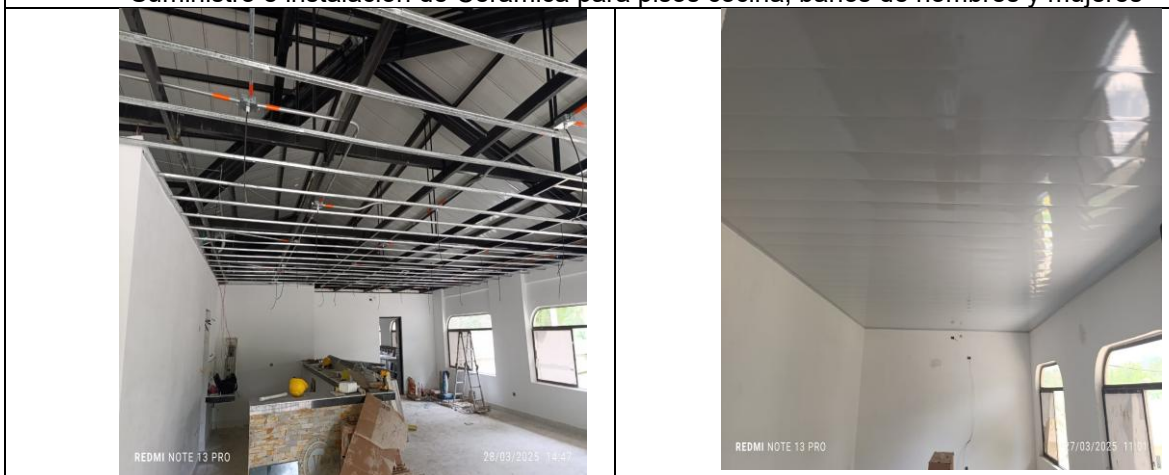
Suministro CIELO RASO SUSPENDIDO PVC casino de oficiales
