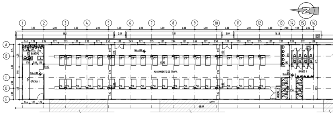
PLANTA GENERAL EXISTENTE Escala: 1:150
