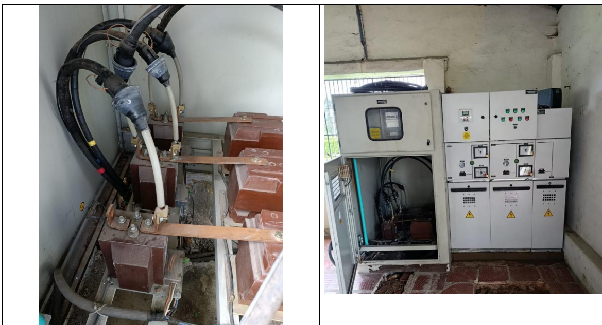
Se realiza conexión, suministro e instalación de terminal - se recibe y ubica celda para conexión y puesta en funcionamiento.
