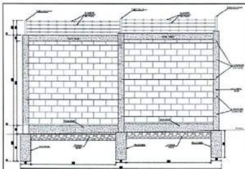
Ilustración 6. Esquema de módulo de cerramiento propuesto – I.E. CODEBAL, Lejanías
